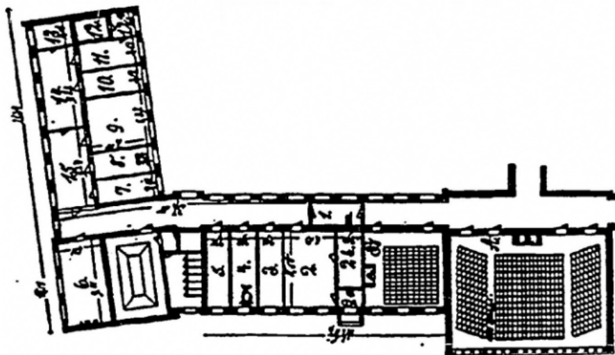
Eksperimentinės psichologijos instituto Leipcigo universitete patalpų planas. 1896 m. Dešinėje – Civinskio minima didžioji auditorija. Šaltinis: W. Wundt. Das Institut für experimentelle Psychologie. Festschrift zur Feier des 500-jährigen Bestehens der Universität Leipzig (Leipzig: Rektor u. Senat der Universität, 1909), vol. 4: Die Institute und Seminare der Philosophischen Fakultät an der Universität Leipzig. 1. Die philosophische und die philosophisch-historische Sektion, 118–133; 123. Autorės dėkoja kolegai David Kent Robinson už sudarytą galimybę publikuoti šią iliustraciją.
