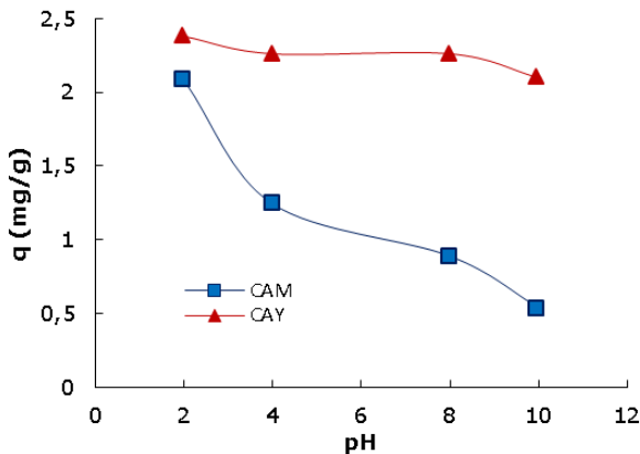
Figura 3. Efecto del pH sobre la capacidad máxima de adsorción.
