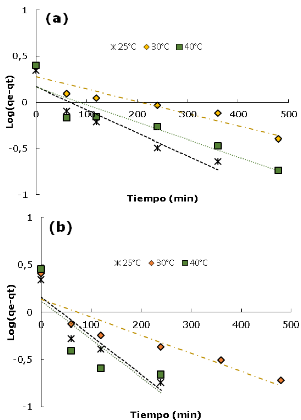
Figura 5. Modelo cinético pseudo primer orden para la adsorción del colorante DB-86 a diferentes temperaturas: a) CAM y b) CAY.
