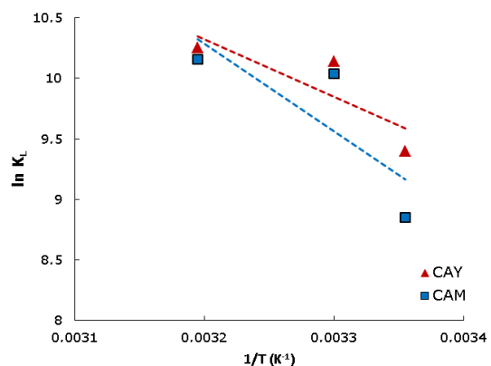
Figura 4. Termodinámica de la adsorción del colorante DB-86 sobre los carbones activados CAY y CAM a pH 2.
