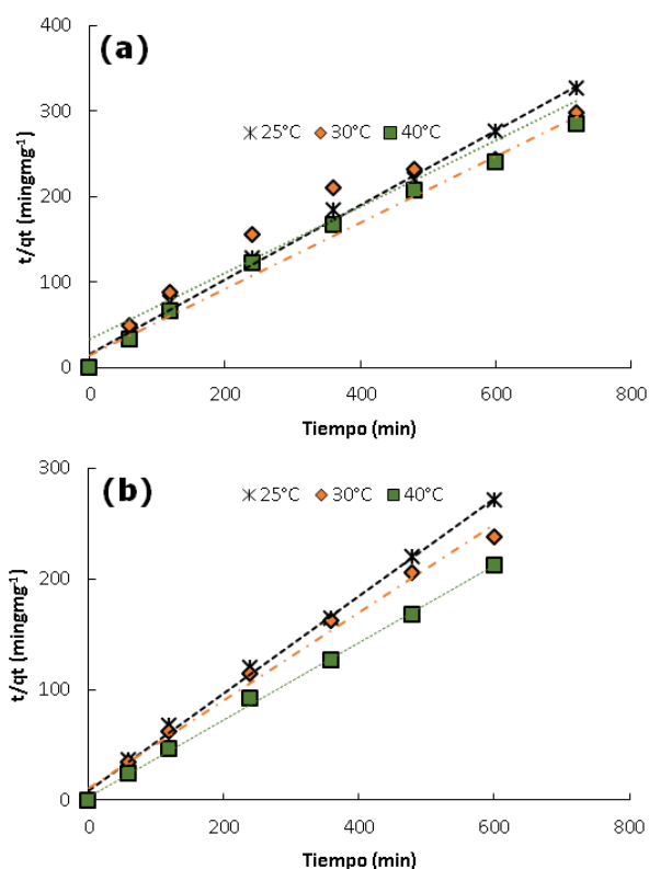
Figura 6. Modelo cinético pseudo segundo orden para la adsorción del colorante DB-86 a diferentes temperaturas: a) CAM y b) CAY.
