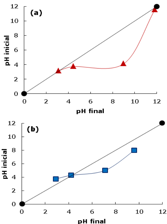
Figura 2. Punto de carga cero del CAY (a) y CAM (b).
