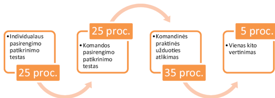
4 pav Siūlomos užduočių atlikimo vertinimo proporcijos parengta autorių
