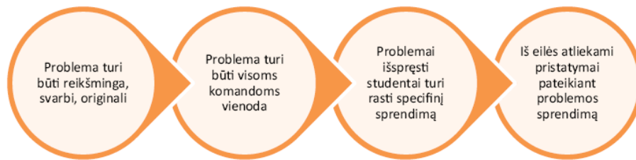
3 pav Praktinių situacijų formavimo ir sprendimo žingsniai parengta autorių
