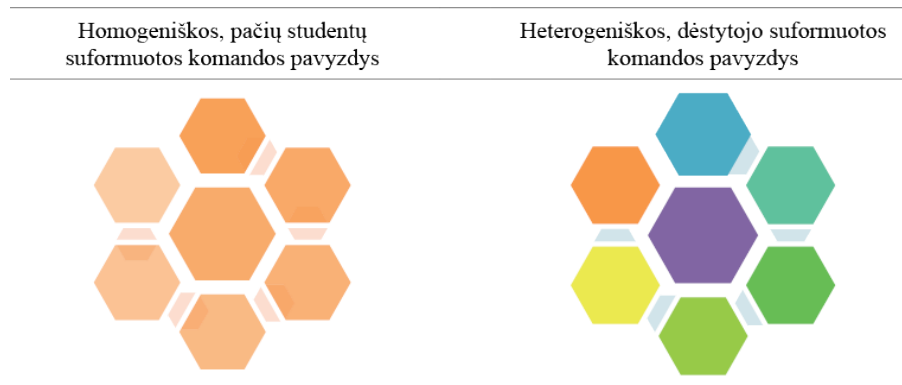
2 pav Komandų formavimo pavyzdžiai parengta autorių
