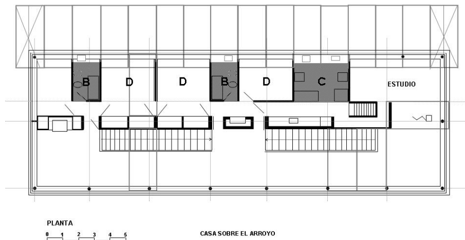
Figura 17 Proporciones y organización en planta de la Casa sobre el Arroyo Dibujo: Carlos Pantaleón
