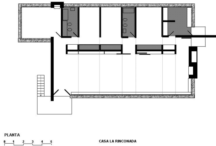
Figura 5 Casa La Rinconada (1945–1948), Punta Ballena, departamento de Maldonado, Uruguay. Arq. Antonio Bonet. Dibujo: Carlos Pantaleón (restitución a partir de diferentes fuentes)
