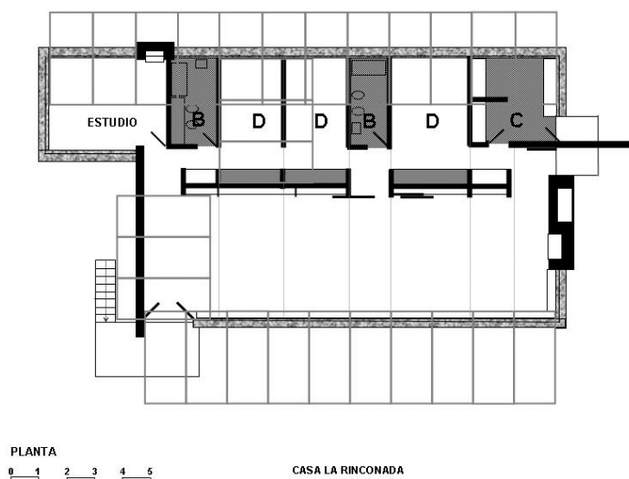
Figura 18 Proporciones y organización en planta Casa La Rinconada Dibujo: Carlos Pantaleón
