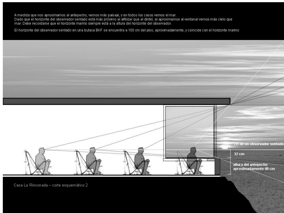
Figura 16 Casa La Rinconada corte esquemático 2 y cálculo del campo visual Dibujo: Carlos Pantaleón
