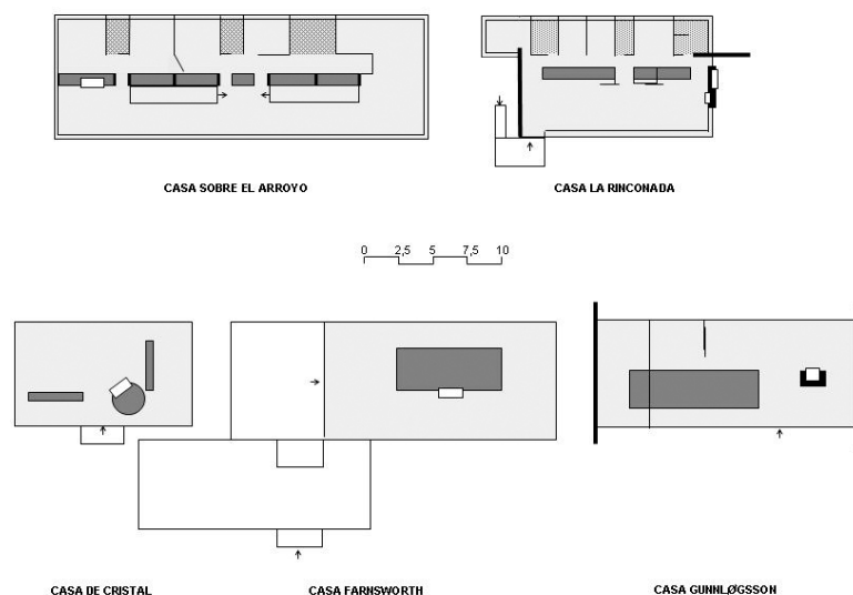
Figura 6. Imágenes de las plantas de las viviendas comparadas. Plantas esquemáticas de las cinco viviendas analizadas a la misma escala. Dibujo: Carlos Pantaleón.
