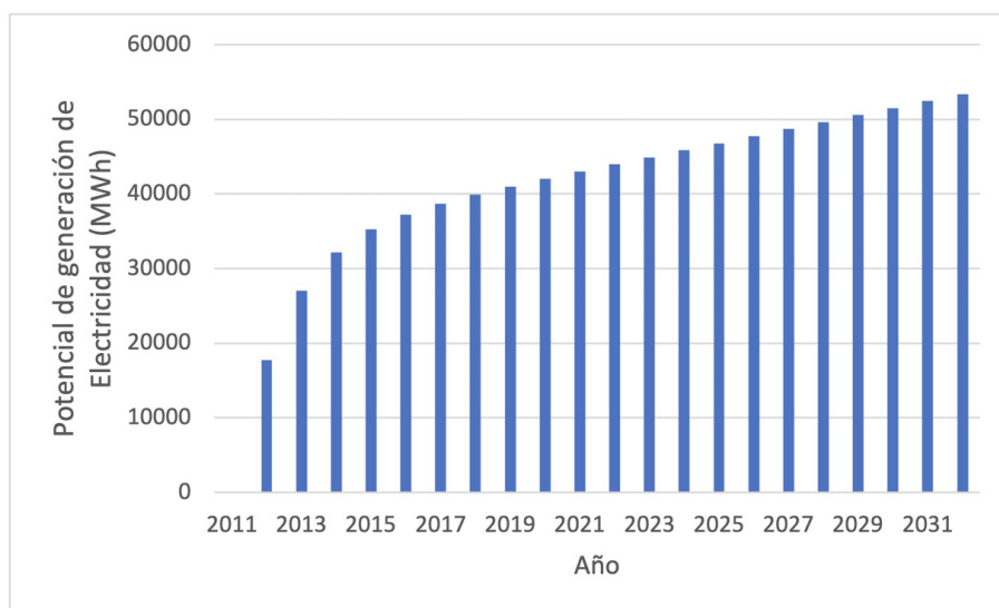
FIGURA 4 Potencial de generacion de electricidad MWh de las fracciones de residuos depositadas en el relleno sanitario mancomunidad PatatePelileo
