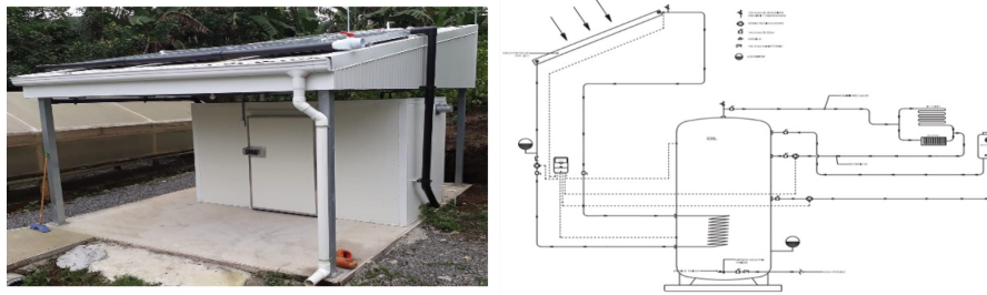
FIGURA 4 Fotografía (izquierda) y esquema (derecha) del prototipo de secador solar activo híbrido forzado implementado en el Tanque de la Fortuna [23]
