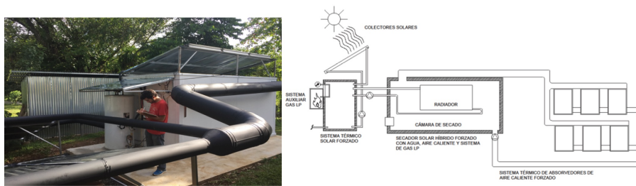
FIGURA 2 Fotografía (izquierda) y esquema (derecha) del prototipo de secador solar activo híbrido forzado implementado en Guatuso. [21]
