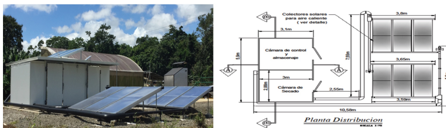
FIGURA 3 Fotografía (izquierda) y esquema (derecha) del prototipo de secador solar activo híbrido forzado implementado en CLSC-ITCR [20]
