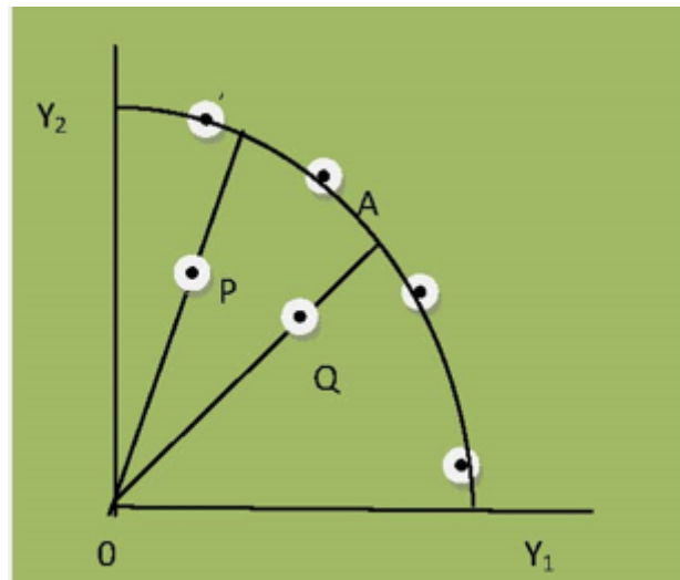
Figura 1 Outputorientado DEA
