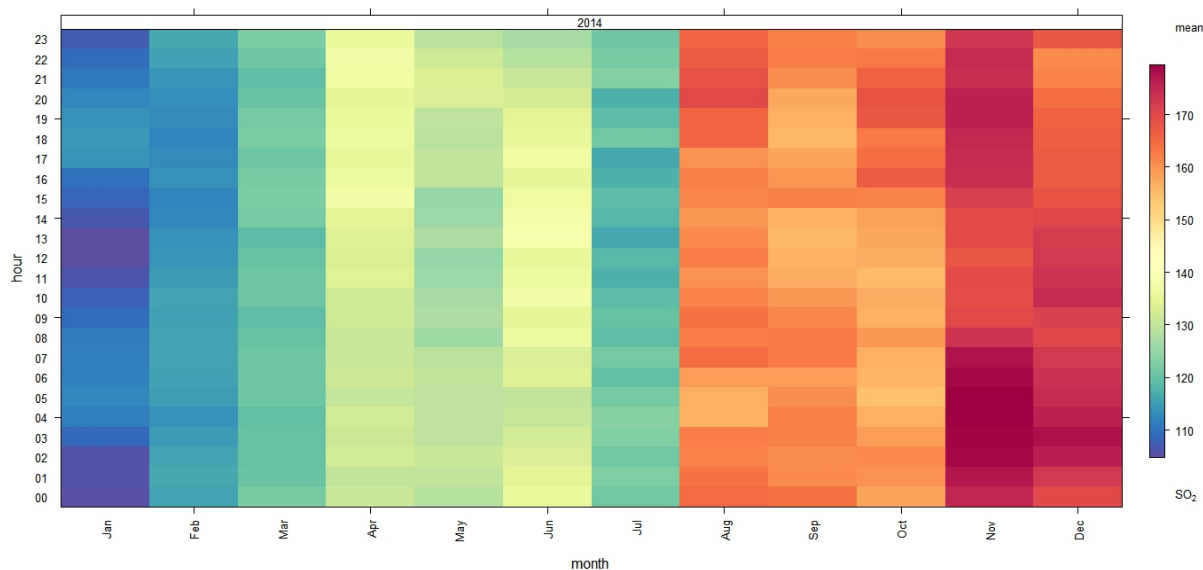
Figura 5. Gráfico de tendencias para el SO 2 en el 2014.
