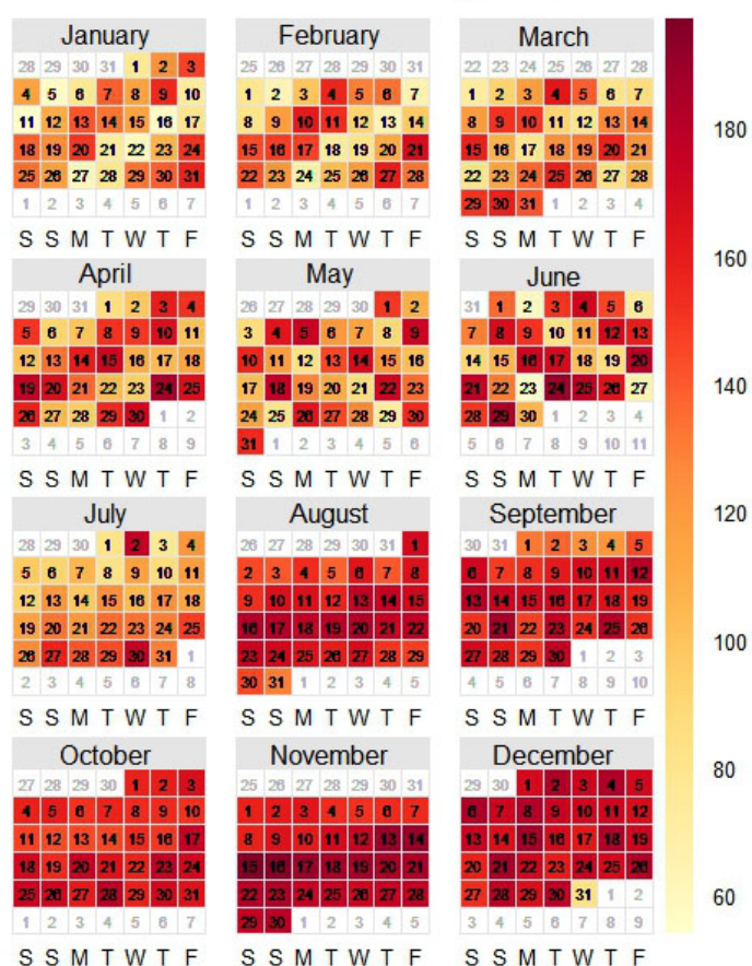
Figura 1. Evolución diaria del SO 2 en 2014
