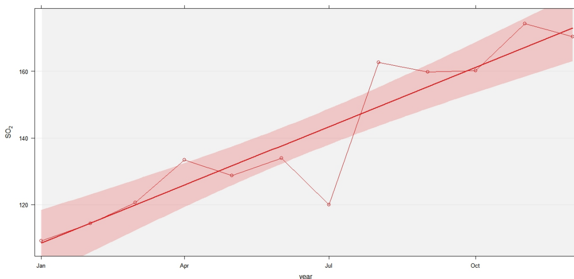
Figura 6. Media mensual de SO 2 en el 2014.
