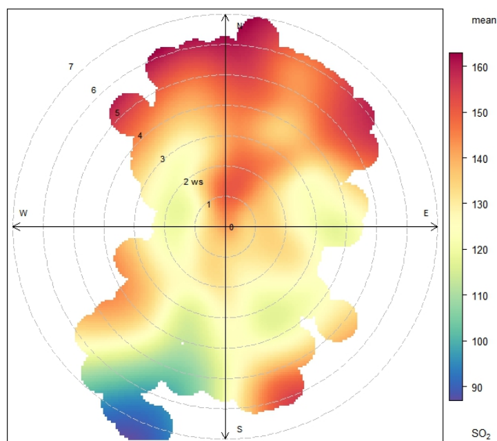
Figura 2. Distribución de medias de SO 2 .
