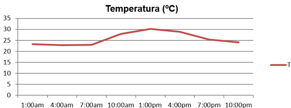
Figura 4. Marcha diaria de la temperatura
