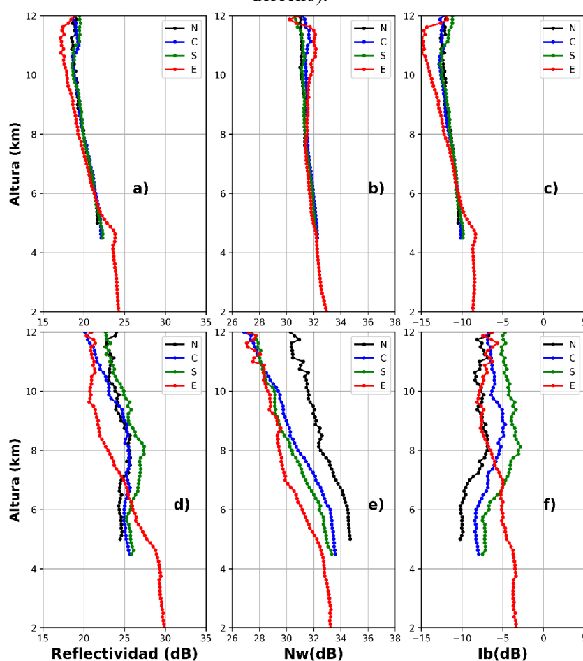
Figura 10. Perfil vertical promedio de la reflectividad y sus componentes determinado desde KuPR-GPM (2014-2018). (a) Reflectividad para lluvia estratiforme (b) Nw para lluvia estratiforme, (c) Ib para lluvia estratiforme, (d) reflectividad para lluvia convectiva (e) Nw para lluvia convectiva y (f) Ib para lluvia convectiva.
