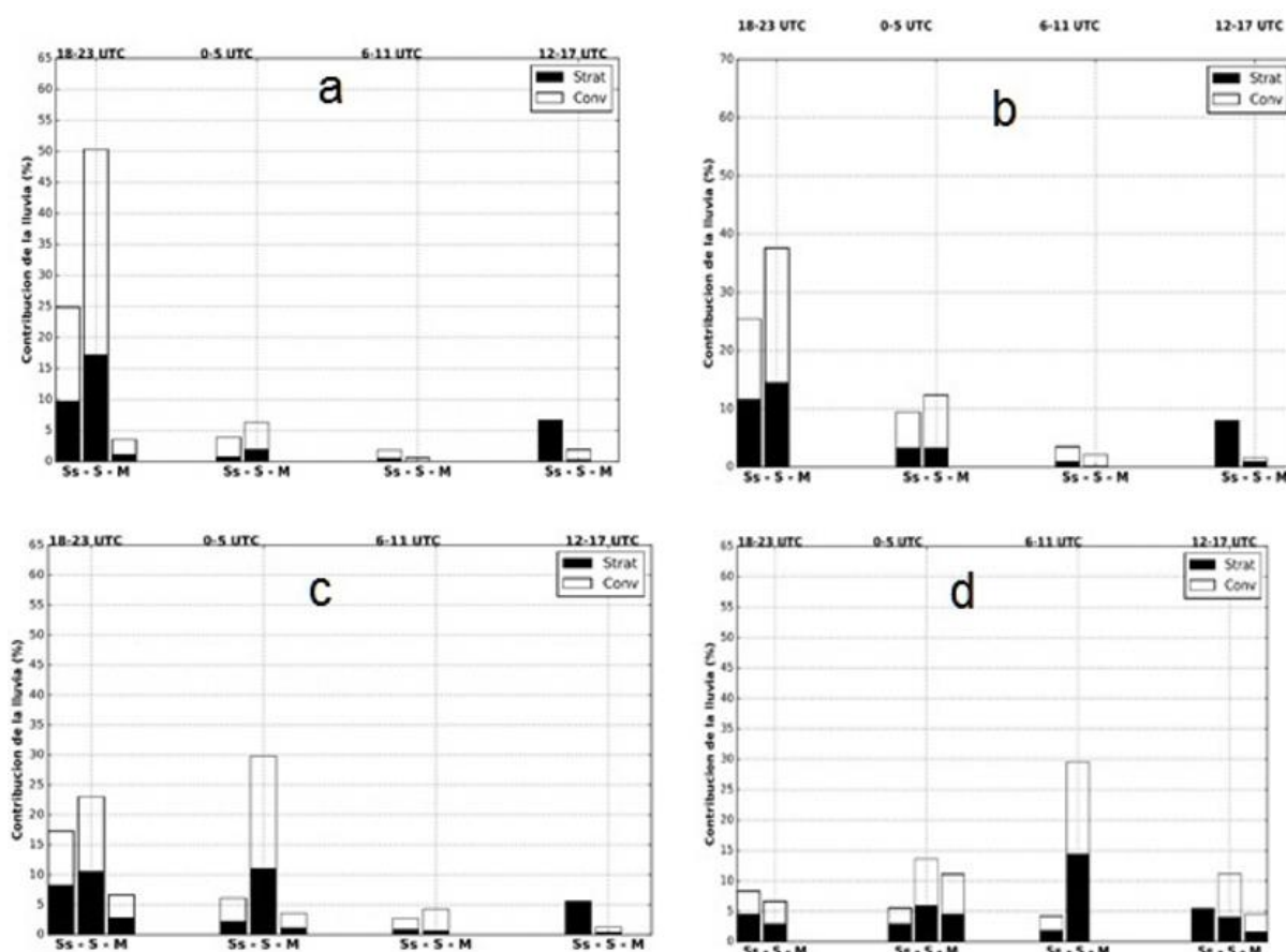
Figura 2. Ciclo diurno de la precipitación y la contribución relativa (%) a la lluvia acumulativa según el tipo de precipitación (convectiva y estratiforme). Determinado desde PR-TRMM y KuPR-GPM de periodo 1998-2018 para la estación lluvioso DJF (diciembre-enero-febrero). a) Región N (panel superior izquierda), b) región C (panel superior derecha), c) región S (panel inferior izquierda) y d) región E (panel inferior derecha).
