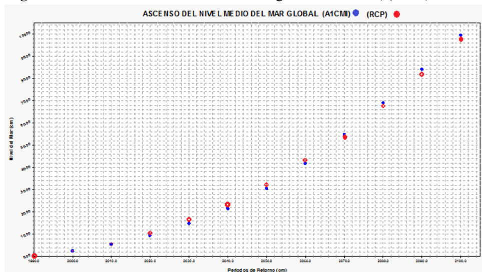
Figura 7. Ascenso del nivel medio del mar global para los escenarios A1CMI y RCP8.5
