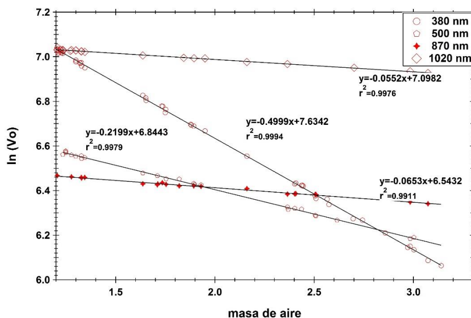
Figura 2. Método Langley para los canales del Microtops II
