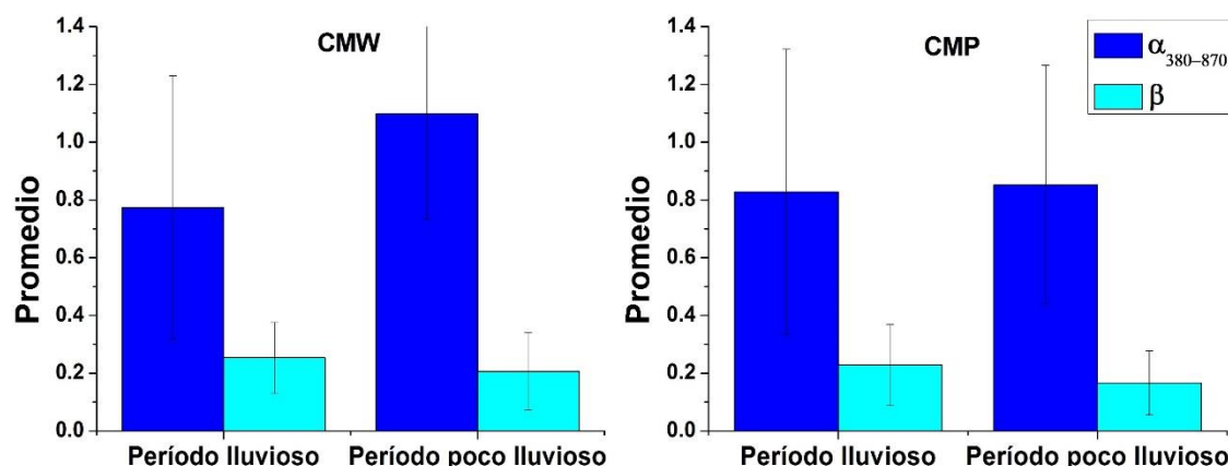
Figura 5. Variación media del \alpha_{380-870} y de \beta durante los periodos lluvioso y poco lluvioso en a) ciudad de Camagüey y b) Centro Meteorológico Provincial.
