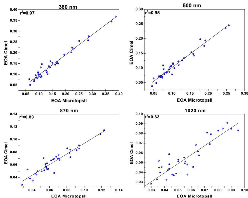
Figura 3. Comparación de los datos del MicrotopsII y el CIMEL.
