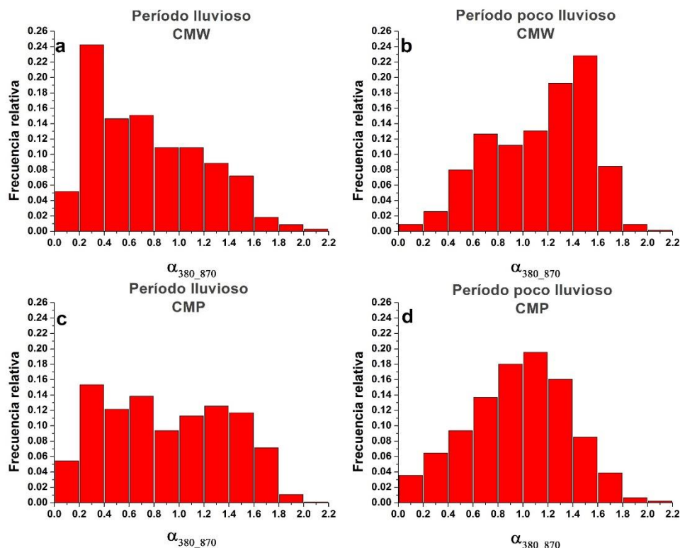
Figura 7. Distribución de frecuencias del \alpha_{380-870} durante el periodo lluvioso en a) CMW y c) CMP y durante el periodo poco lluvioso en b) CMW y d) CMP.
