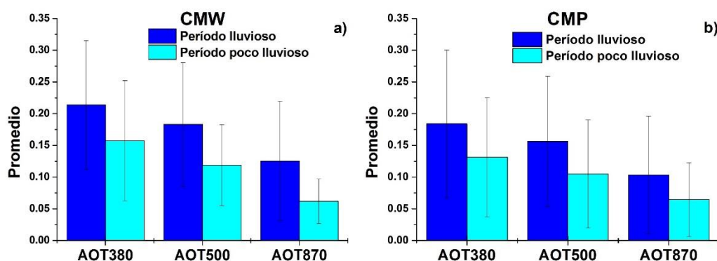
Figura 4. Variación espectral media del espesor óptico de los aerosoles durante los períodos lluvioso y poco lluvioso en a) ciudad de Camagüey y b) Centro Meteorológico Provincial.
