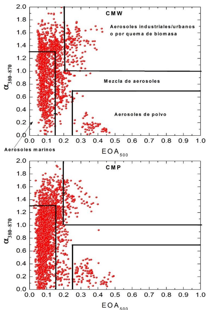
Figura 8. Diagrama de dispersión de \alpha_{380-870} y del EOA_{500} para la discriminación de los diferentes tipos de aerosoles
