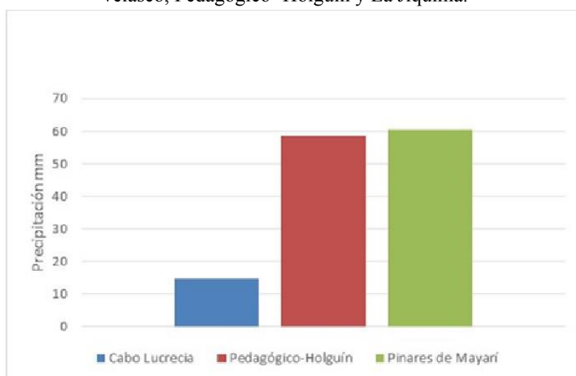
Figura 6. Error absoluto para el acumulado anual de precipitación durante el año 2016.
