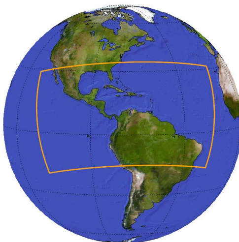
Figura 1. Dominio regional de CAMC definido en CORDEX (contorno rojo) . Tomado de http://cordex.org/wp-content/uploads/2012/11/images_pdf_documentation_CORDEX_domain_description_230615.pdf
