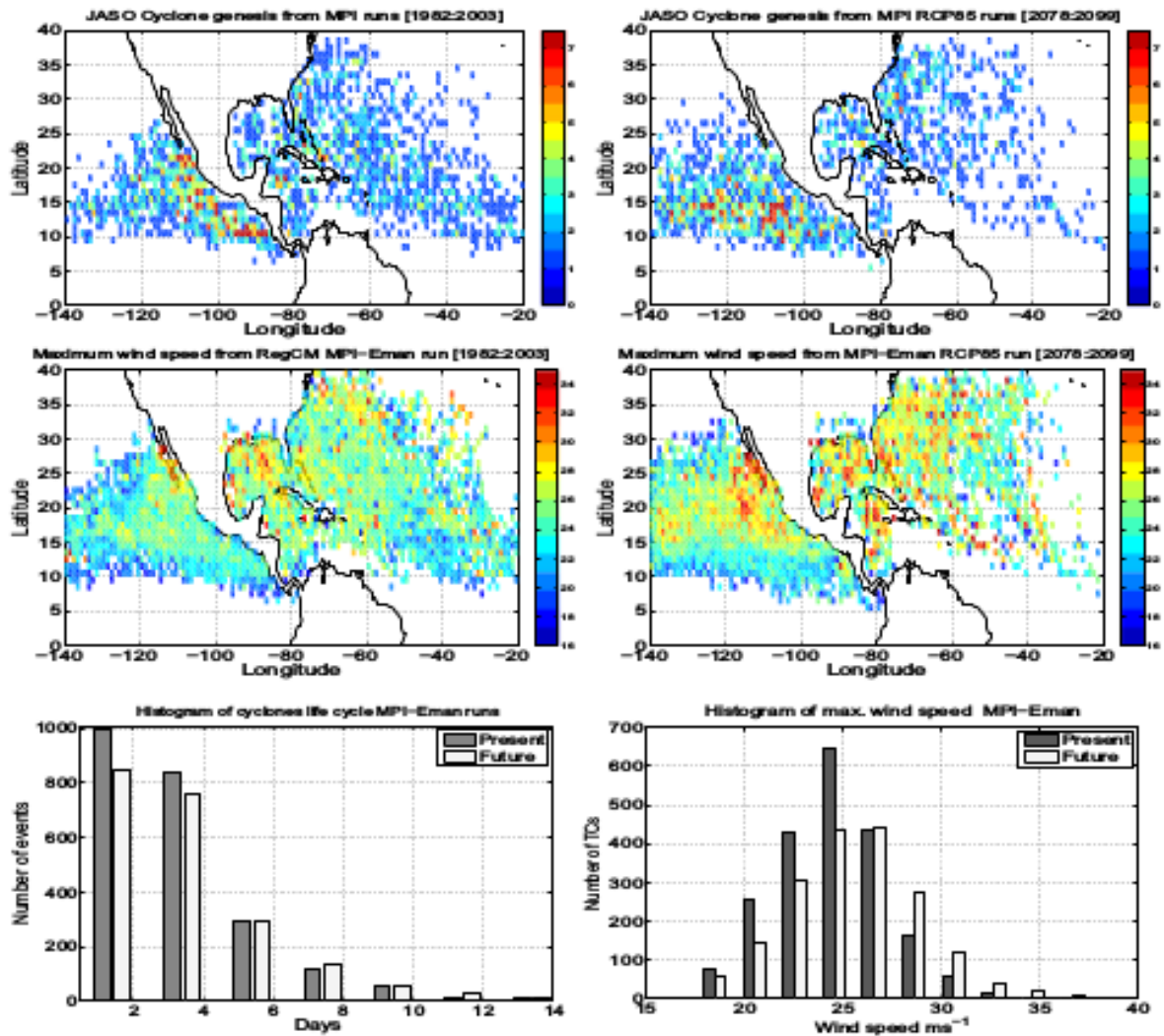
Figura 9. Características de CT en el 2078-2099 relativas a 1982-2003. (Tomado de Diro et al. 2014 )
