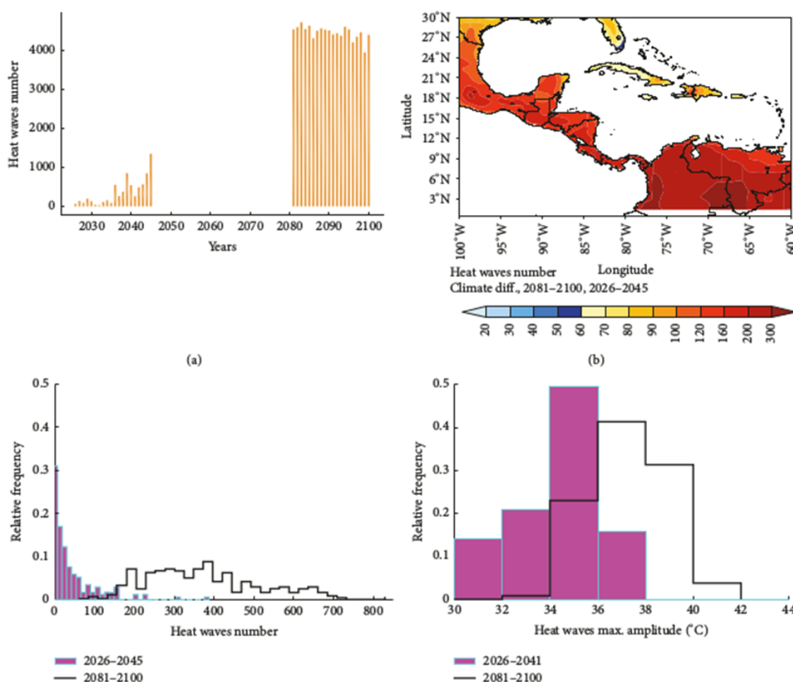
Figura 7. Media del conjunto multimodelo para el escenario de RCP8.5: (a) series temporales anuales, (b) cambio de número de olas de calor entre los períodos climáticos 2081-2100 y 2026-2045, (c) frecuencia de olas de calor de toda la región, incluida la zona oceánica, y (d) promedio regional de olas de calor de amplitud máxima. (Tomado de Ángeles-Malaspina et al. 2018 )
