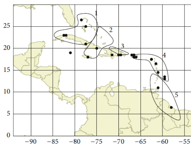
Figura 5. Zonas definidas en el trabajo de McLean et al (2015) para las proyecciones de los parámetros relacionados con extremos de temperatura y lluvia. (Tomado de McLean et al., 2015 )
