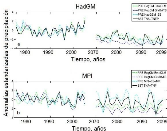
Figura 4. Series temporales de anomalías estandarizadas de precipitación y del gradiente de TSM ANT-PNT para el período de verano (JJAS) sobre CAMM para las salidas del RegCM4 con condiciones de contorno de los MCG HadCM (a) y MPI (b) para los períodos de referencia y de fines del siglo (Adaptado de Fuentes-Franco et al., 2014)
