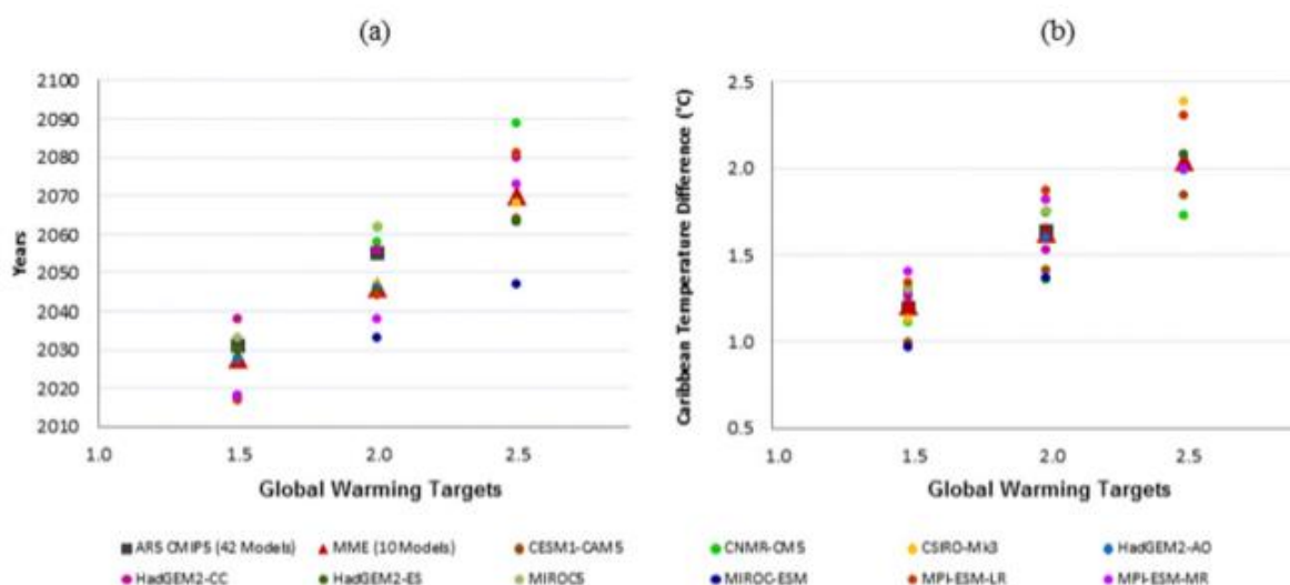
Figura 10. a) Años proyectados por los 10 modelos para los tres objetivos de calentamiento global (1.58, 2.08 y 2.58°C). (b) promedio anual del Caribe anomalías de temperatura (8C) con respecto a la línea de base preindustrial proyectada por los 10 modelos para los tres objetivos de calentamiento global. (Tomado de Taylor et al., 2018 )
