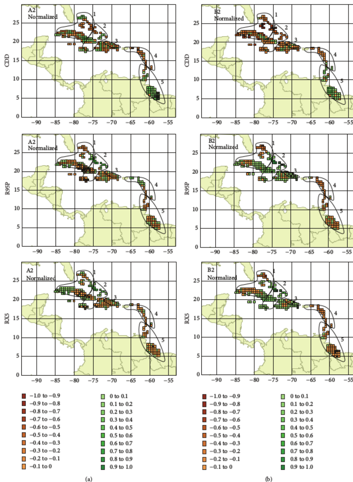
Figura 6. Cambios normalizados proyectados en las tendencias para DDC, R95P y RX5 para 2071-2099 en relación con 1961-1989 para A2 (paneles izquierdos) y B2 (paneles de la derecha) Escenarios IPCC SRES. (Tomado de McLean et al., 2015 )
