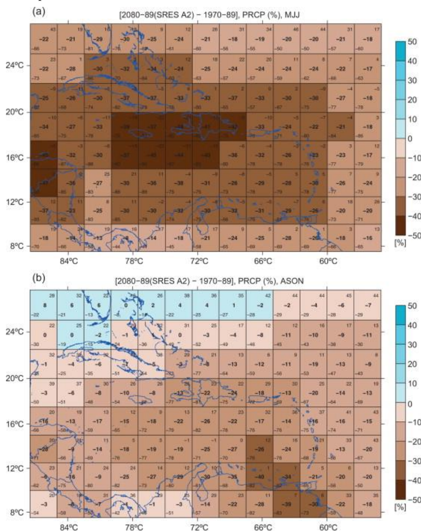
Figura 3. Cambio proyectado en la precipitación (%) para el 2080 en el escenario SRES A2 basado en el CMIP3. (Tomado de Karmalkar et al. 2013 )
