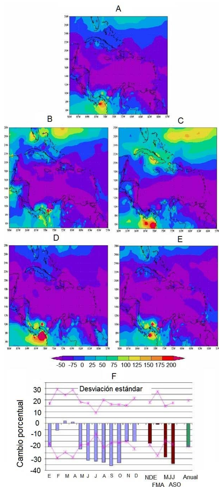
Figura 2. Proyecciones de precipitaciones para el período 2071-2100 relativas al período de referencia de 1961-1990, bajo el escenario A2 (Cambio porcentuales) Los paneles (A), (B), (C), (D) y (E) representan la precipitación anual, y los trimestres NDE, FMA, MJJ y ASO, respectivamente. El panel (F) muestra los cambios mensuales, trimestrales y anuales calculados promediando el dominio mostrado en A-E. La línea continua representa una desviación estándar calculada del conjunto de salidas de CMAP. (Tomado de Campbell et al. 2010 )
