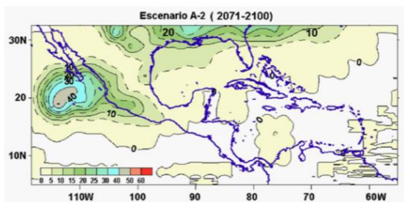
Figura 8. Isolíneas de densidad de trayectorias de vórtices representativos de ciclones tropicales obtenidas de la salida del sistema de modelación climática PRECIS obtenida para el periodo 2071-2100 con las condiciones de concentración de CO 2 del escenario SRES-A2 y con las condiciones de frontera de la salida del HadCM3 correspondiente a dicho escenario. (Tomado de Martínez-Castro et al., 2011 )
