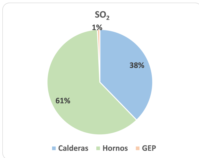
Figura 5. Proporción relativa de las emisiones de \text{SO}_2 en la provincia Cienfuegos por tipo de fuente.
