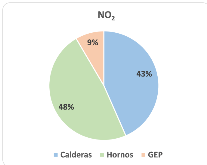
Figura 6. Proporción relativa de las emisiones de \text{NO}_2 en la provincia Cienfuegos por tipo de fuente.
