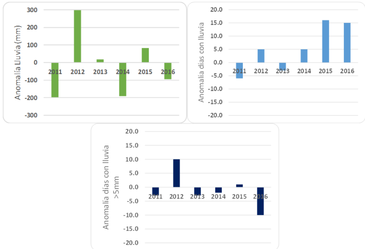
Figura 7. Comportamiento de las anomalías de las precipitaciones, días con lluvias y días con lluvias >5mm.
