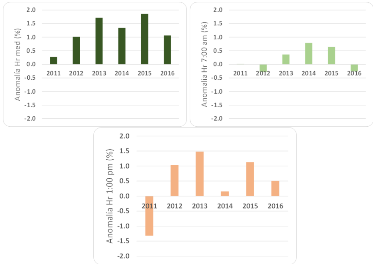
Figura 8. Comportamiento de las anomalías de la humedad relativa.
