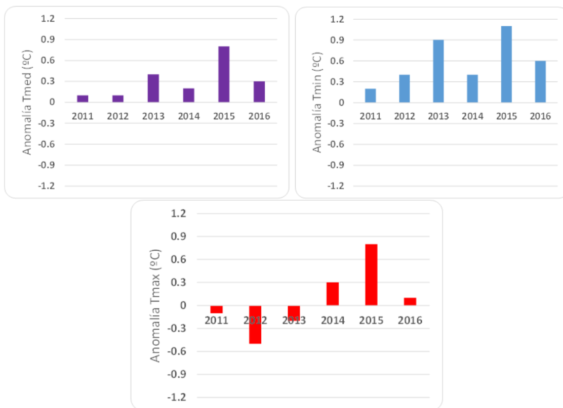
Figura 5. Comportamiento de las anomalías de las temperaturas: media, mínima y máxima.
