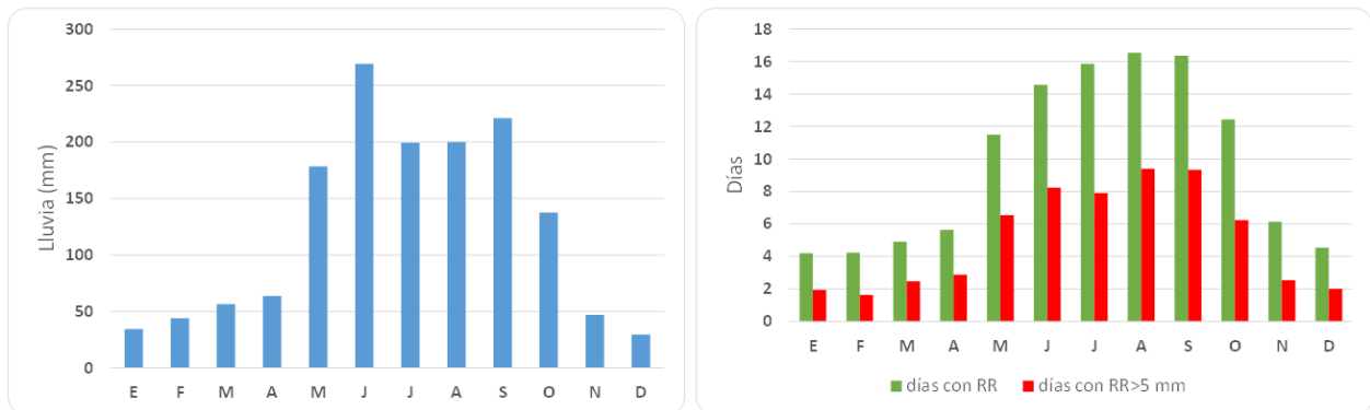
Figura 3. Comportamiento de las precipitaciones (izquierda), los días con lluvias (días con RR) y días con lluvia >5 mm (días con RR>5 mm) en Aguada de Pasajeros en el período 1981-2010.
