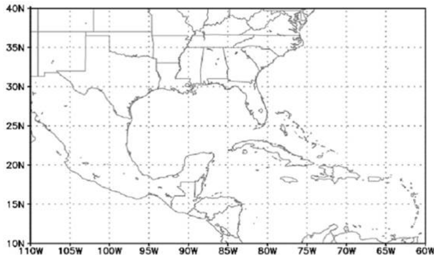
Figura 2. Región sinóptica empleada
