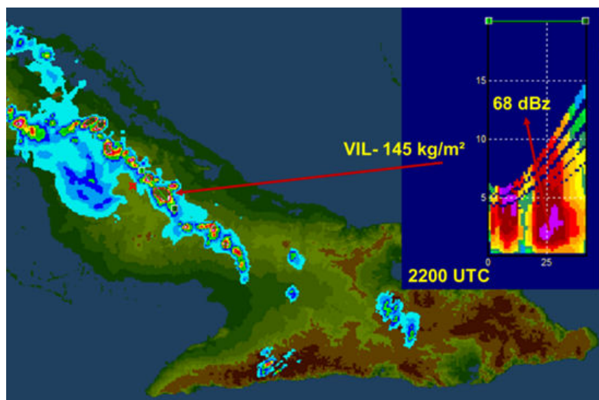
Figura 6. Corte vertical que muestra los altos valores de VIL y el eco de máxima reflectividad por debajo de los 5 km, el 2 de julio de 2014 en Camagüey
