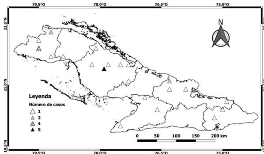
Figura 1. Distribución de los casos de TLS que generaron lluvias localmente intensas.
