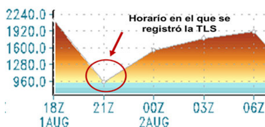
Figura 9. Meteograma que muestra la disminución de la altura del NCA en el horario cercano al que ocurrió la TLS, para el día 1/8/2015 en la estación meteorológica de Florida, Camagüey.
