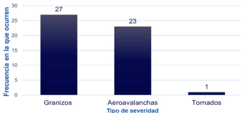
Figura 3. Comportamiento del tipo de severidad manifestado en las tormentas locales que generaron lluvia intensa
