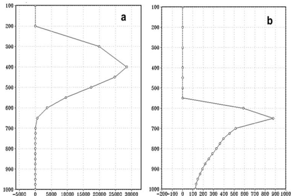
Figura 11. Corte vertical del contenido de granizo (a) y el contenido de lluvia (b) el 1/8/2015 a las 2100 UTC en la estación meteorológica de Florida, Camagüey
