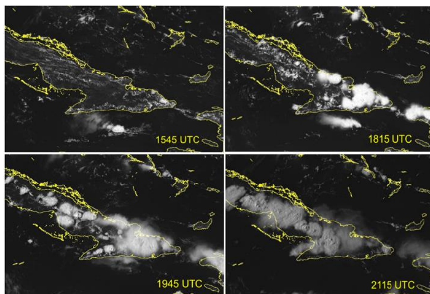
Figura 5. Secuencia de imágenes de satélite GOES 13, del día 13 de agosto de 2015 donde se observa la formación de actividad convectiva fuerte
