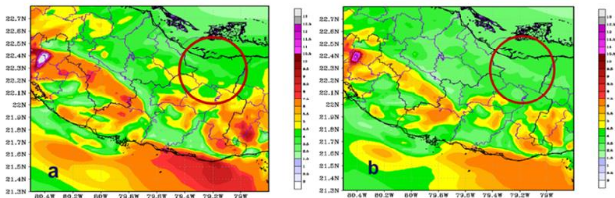
Figura 12. Comportamiento de la cizalladura vertical (a) en la capa superficie- 850 hPa (b) en la capa superficie- 700 hPa, en el municipio de Yaguajay el 29/5/2016
