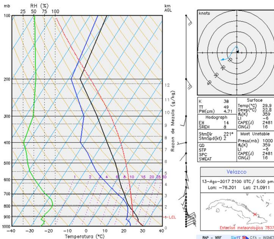
Figura 10. Sondeo del día 13 de agosto de 2017 en la estación meteorológica de Velasco, Holguín a las 2100 UTC
