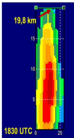
Figura 7. Corte vertical del día 24 de julio de 2017 en Niquero, Granma que muestra el tope alcanzado por la TLS generadora de lluvia intensa
