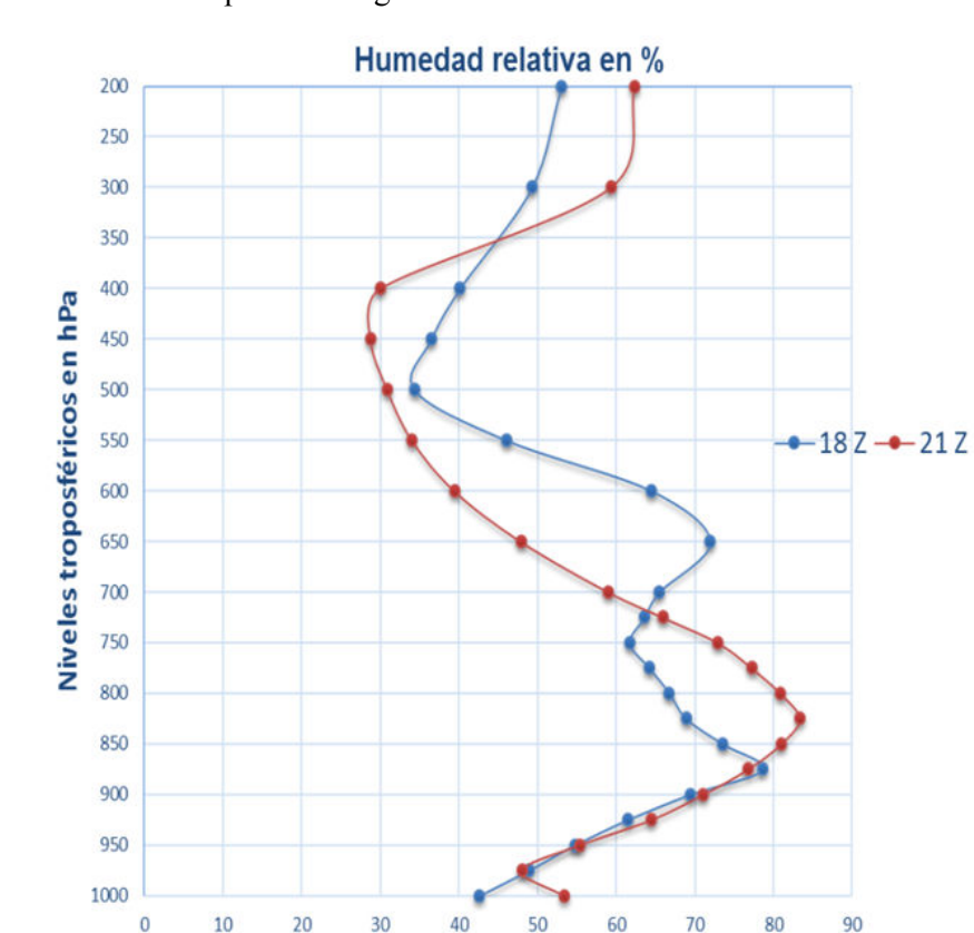
Figura 8. Comportamiento de la humedad relativa a las 1800 UTC y a las 2100 UTC del día 13/8/2017 en Velazco, Holguín
