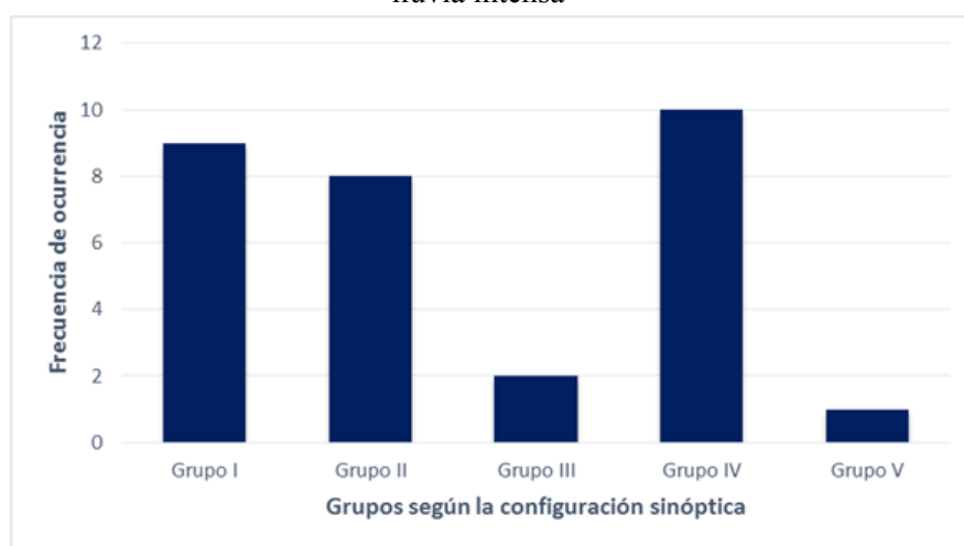
Figura 4. Distribución de los casos según la configuración sinóptica en la que se desarrollaron
