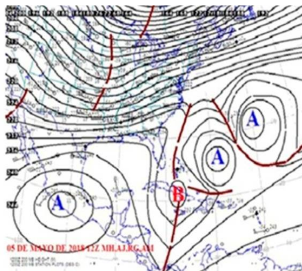
Figura 3. Altura geopotencial en el nivel de 200 hPa del día 5 de mayo del 2018 en el horario de las 1200 UTC
