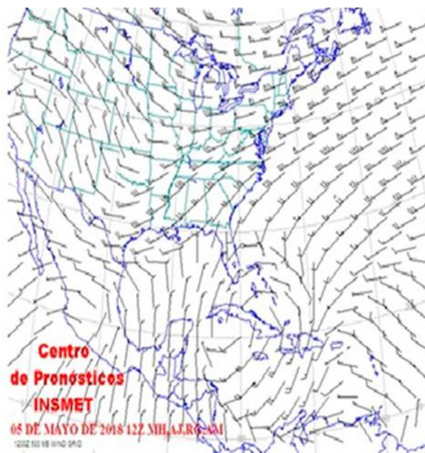
Figura 5. Flujo del viento en el nivel 500 hPa en el horario de las 1200 UTC
