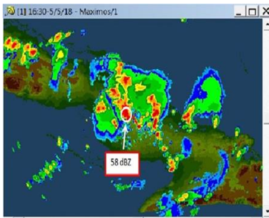
Figura 8. Imagen obtenida por el radar meteorológico de Camagüey del día 5 de mayo del 2018 a las 16:30 hora local.
