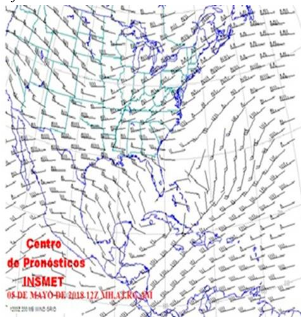
Figura 6. Flujo del viento en el nivel 200 hPa a las 1200 UTC
