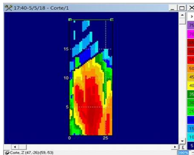
Figura 11. Corte Vertical realizado en el horario de las 17:40 hora local por el radar de Camagüey Master en Ciencias Meteorológicas. La Habana, Cuba.
