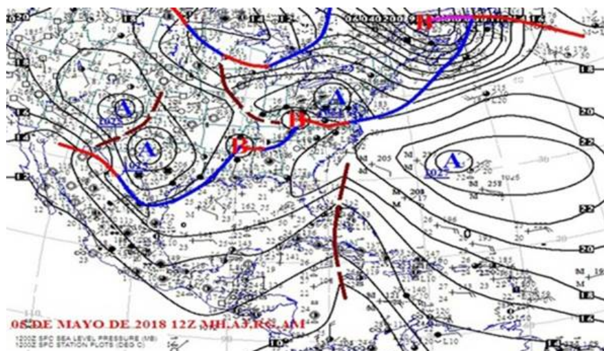
Figura 1. Mapa Sinóptico de superficie del día 5 de mayo 2018 en el horario de las 1200 UTC
