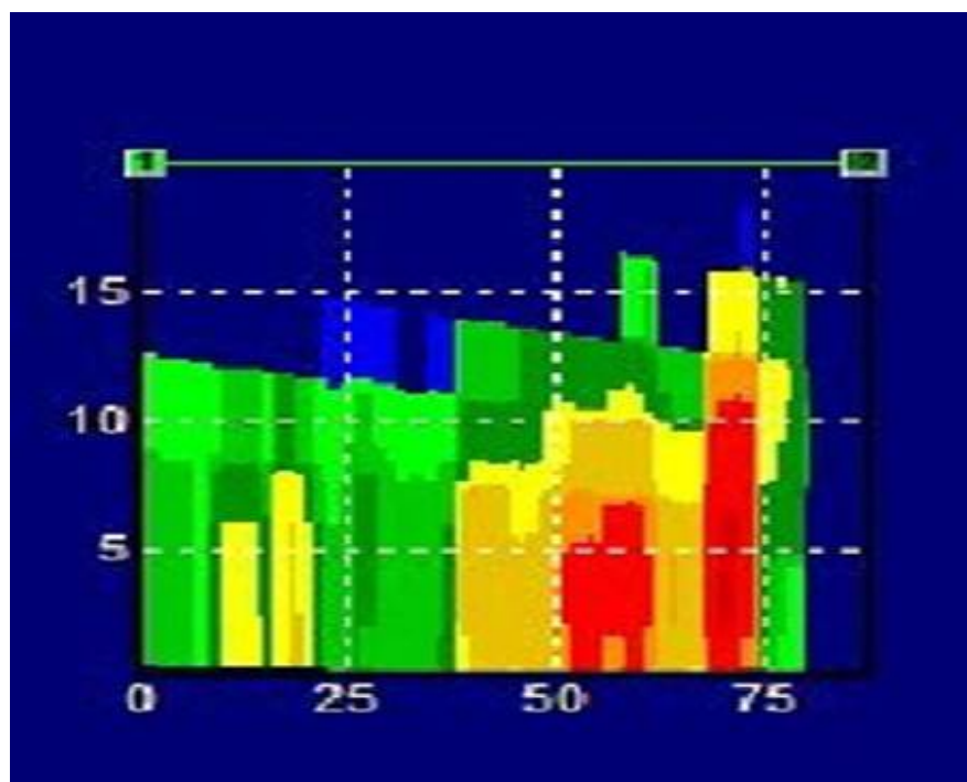
Figura 9. Corte Vertical realizado en el horario de las 16:30 hora local con el radar de Holguín.
