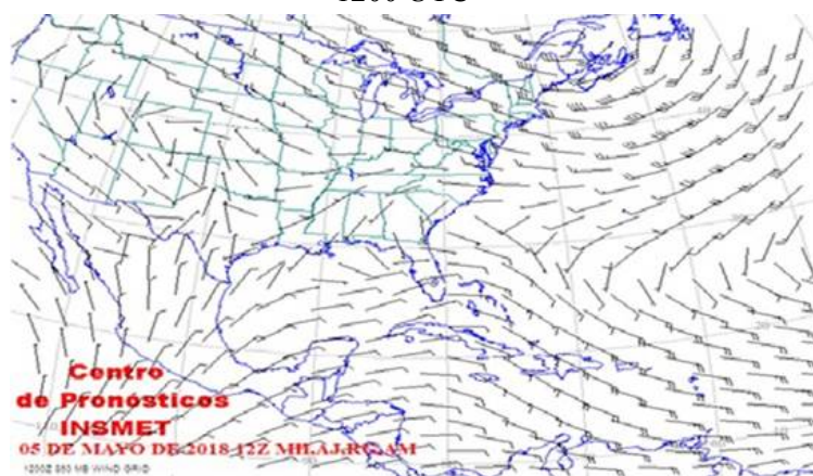
Figura 4. Flujo del viento en el nivel 850 hPa en el horario de las 1200 UTC
