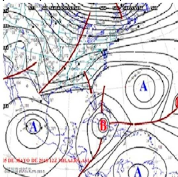
Figura 2. Altura geopotencial en los 500 hPa del día 5 de mayo del 2018 en el horario de las 1200 UTC los niveles hasta 450 hPa están secos y solo se observan que están húmedos entre 900 y 800 hPa
