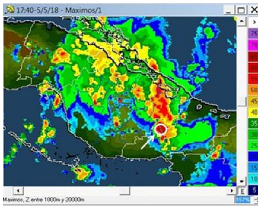
Figura 10. Máxima reflectividad en Guáimaro obtenida por el radar de Camagüey la máxima reflectividad de 66 dBz y un tope de 18 km de altura, que estuvo generada por mecanismos de formación continua de celdas de gran desarrollo. Estas imágenes se realizaron con el radar de Camaguey.
