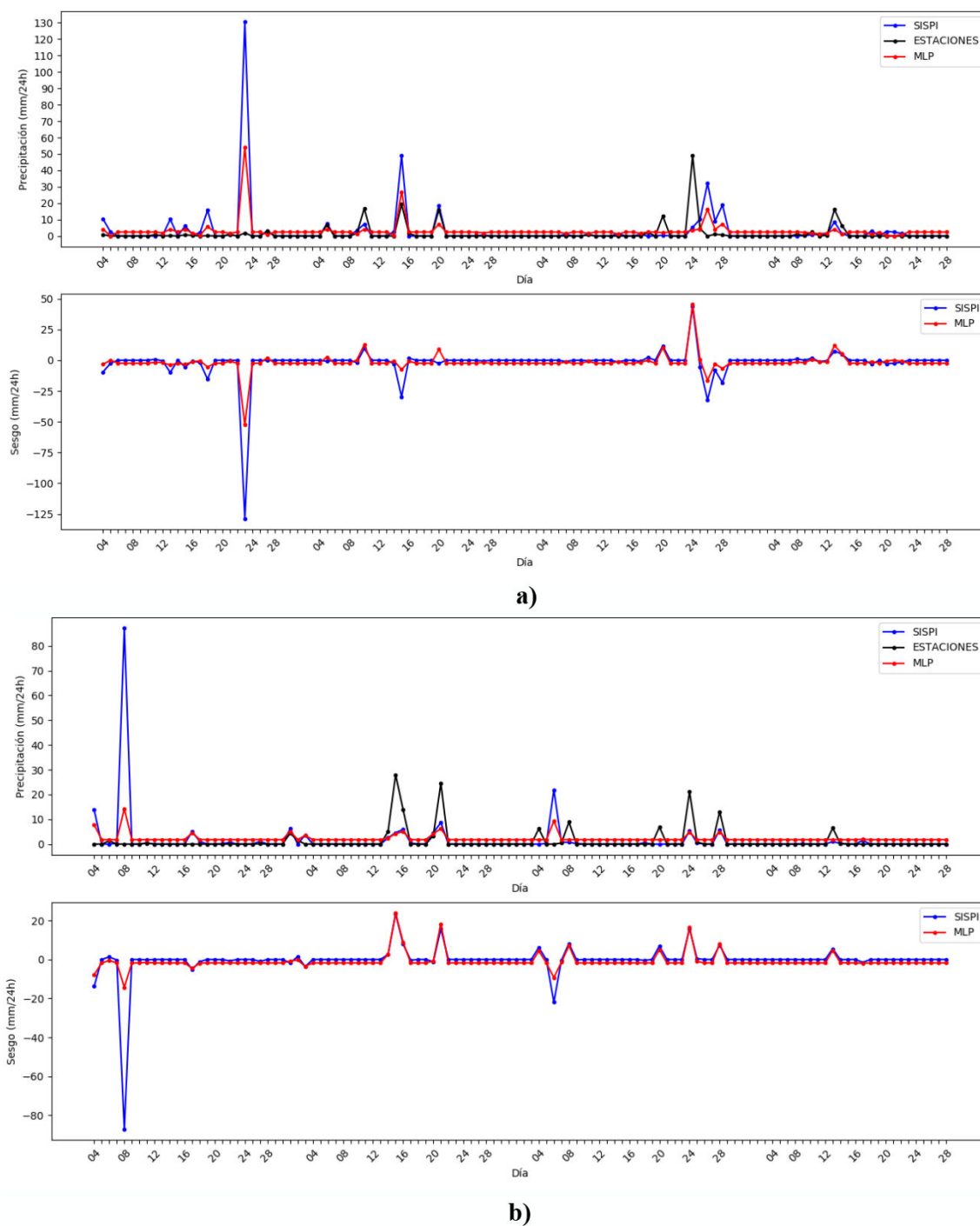
Figura 8. Se muestra el comportamiento del WRF, el MLP y el los valores observados de la precipitación para las estaciones 325 (a) y 333 (b). En el panel superior se muestra el acumulado de precipitación en 24 horas desde el 4 de noviembre de 2018 hasta el 28 de febrero de 2019, se utilizan los colores azul, negro y rojo para el modelo WRF (SisPI), las estaciones (ESTACIONES) y el modelo de red (MLP) respectivamente. En el panel inferior se muestra el sesgo.
