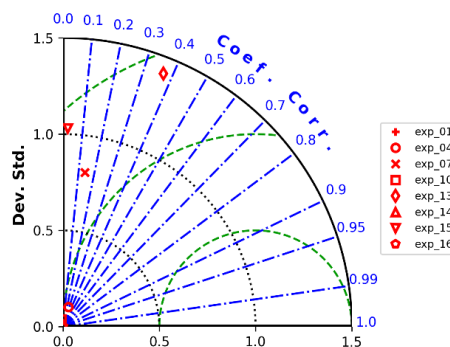
Figura 3. Diagrama de Taylor (333)
