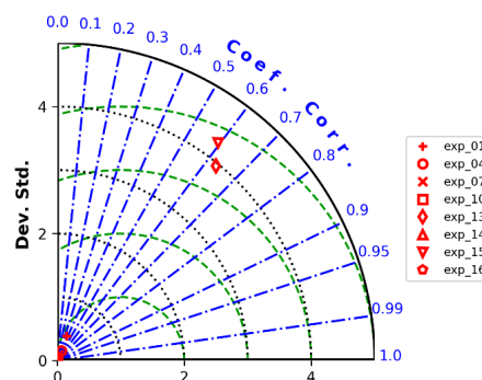
Figura 4. Diagrama de Taylor (342)
