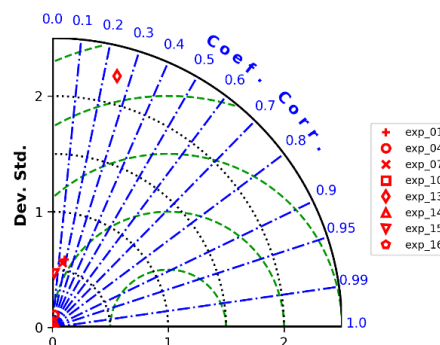
Figura 2. Diagrama de Taylor (325)
