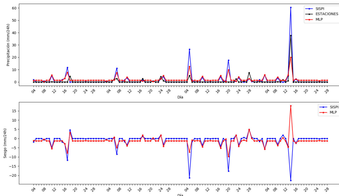
Figura 6. En el panel superior se muestra el acumulado de precipitación en 24 horas desde el 4 de noviembre de 2018 hasta el 28 de febrero de 2019, correspondiente a la estación 355; se utilizan los colores azul, negro y rojo para el modelo WRF (SisPI), las estaciones (ESTACIONES) y el modelo de red (MLP) respectivamente. En el panel inferior se muestra el sesgo.
