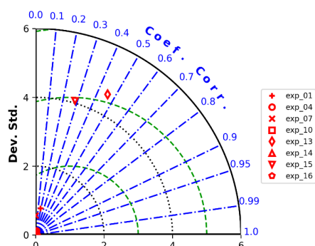
Figura 5. Diagrama de Taylor (355)
