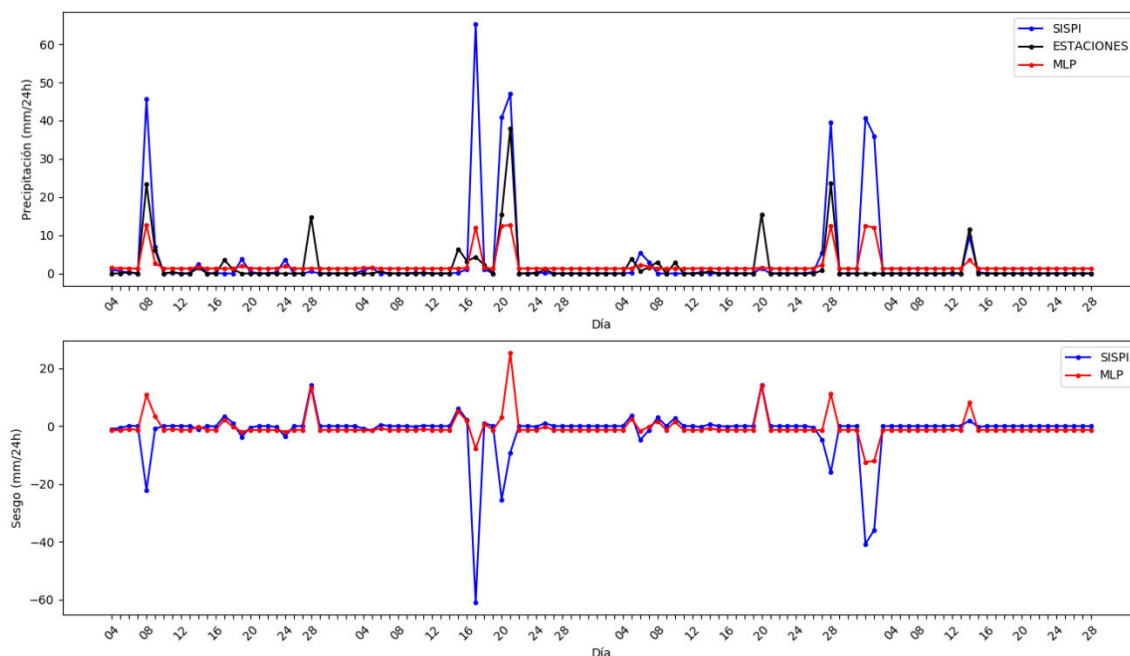
Figura 7. En el panel superior se muestra el acumulado de precipitación en 24 horas desde el 4 de noviembre de 2018 hasta el 28 de febrero de 2019, correspondiente a la estación 342; se utilizan los colores azul, negro y rojo para el modelo WRF (SisPI), las estaciones (ESTACIONES) y el modelo de red (MLP) respectivamente. En el panel inferior se muestra el sesgo.
