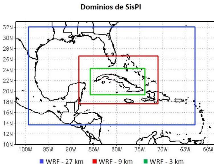
Tomado de (Sierra, et al. , 2014) Figura 1. Dominios del modelo WRF.
