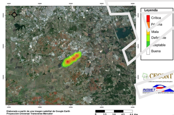
Figura 4. Distribución espacial del ICA, para los promedios anuales de concentraciones de los contaminantes del 2017 al 2019
