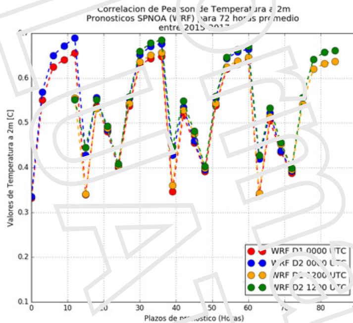
Figura 3.2.3. Correlacion de Pearson de T 2 m
