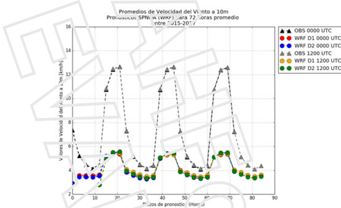
Figura 3.3.1. Promedios de v v 10 m
