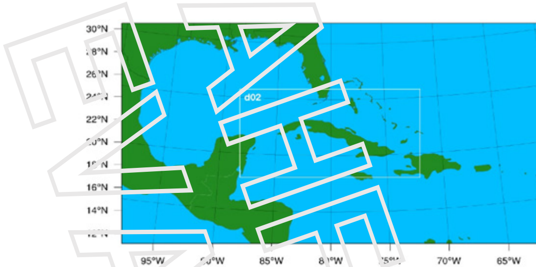
Figura 2.3. Dominios de la configuración del modelo WRF de SPNOA
