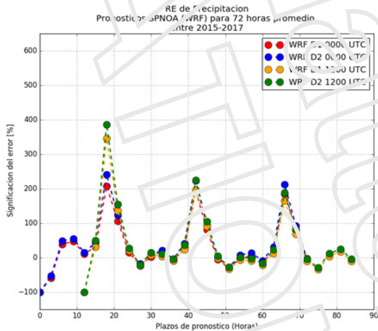
Figura 3.5.3. Error relativo medio de' APS
