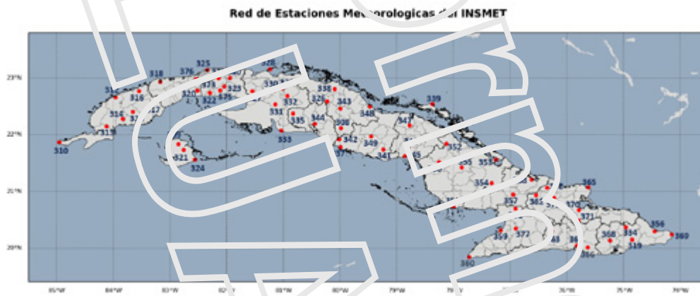
Figura 2.2. Red de estaciones meteorológicas de Cuba
