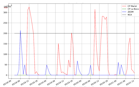
Figura 9. Comportamiento de los receptores discretos para el \text{PM}_{10}
