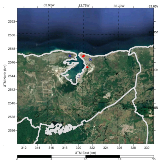
Figura 1. Dominio de la modelación
