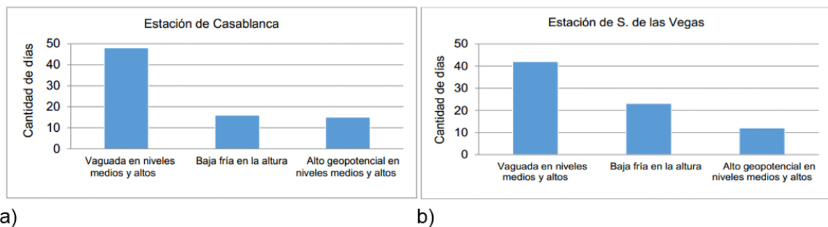
Figura 7. Situaciones predominantes en la altura con influencia anticiclónica en superficie por estación. a) Casablanca, b) Santiago de las Vegas
