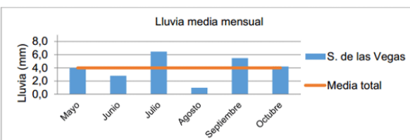
Figura 5. Acumulado medio de lluvia en la mañana por mes por estación. a) Casablanca, b) Santiago de las Vegas
