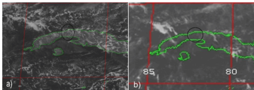
Figura 10. Imagen de satélite: a) Visible, se observa sobre la región de estudio, nubosidad baja proveniente del mar, b) Infrarroja, se observan topes cálidos
