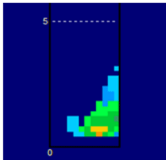
Figura 17. Corte vertical de una celda asociada con el cable de cúmulos formado sobre el estrecho de la Florida
