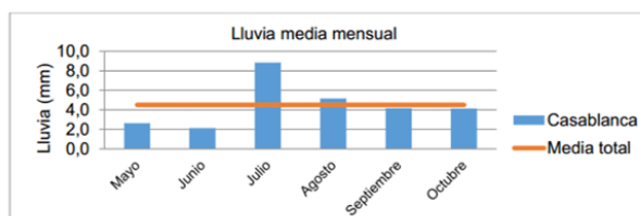
Figura 5. Acumulado medio de lluvia en la mañana por mes por estación. a) Casablanca, b) Santiago de las Vegas
