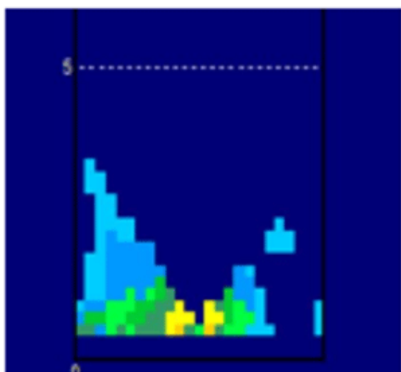
Figura 15. Corte vertical de una celda asociada con los rollos convectivos horizontales
