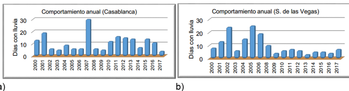
Figura 2. Variabilidad interanual de días con lluvia en la mañana en los períodos lluviosos comprendidos entre 2000-2017 por estación. a) Casablanca, b) Santiago de las Vegas
