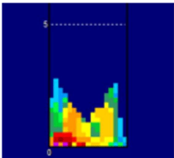
Figura 14. Corte vertical de celdas asociadas con la nubosidad baja proveniente del mar
