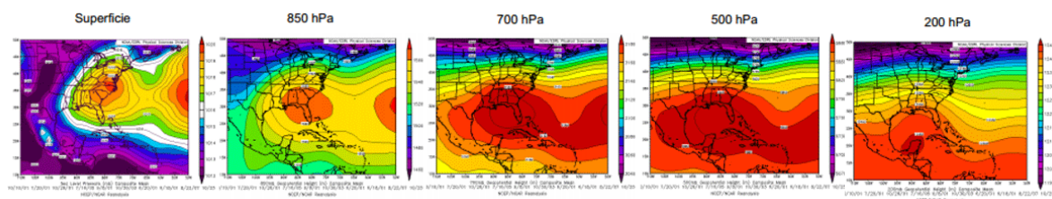
Figura 8. Mapas medios de presión a nivel del mar y niveles troposféricos. Lluvia en la estación de Casablanca
