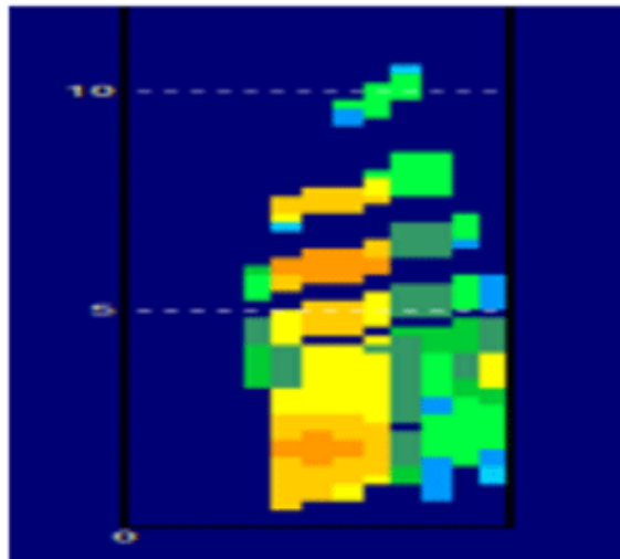
Figura 16. Corte vertical de una celda formada por la convergencia del frente de brisas marinas con los rollos convectivos horizontales
