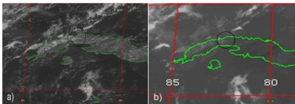
Figura 11. Imagen de satélite: a) Visible, se observa sobre la región de estudio, nubosidad baja asociada con los HCR, b) Infrarroja, se observan topes cálidos
