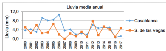
Figura 3. Acumulado medio de lluvia en la mañana por año en las estaciones meteorológicas de La Habana
