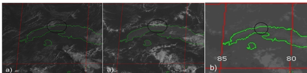
Figura 13. Imagen de satélite: a) Visible, se aprecia el cable en el estrecho de la Florida, b) Infrarroja, se observan topos cálidos
