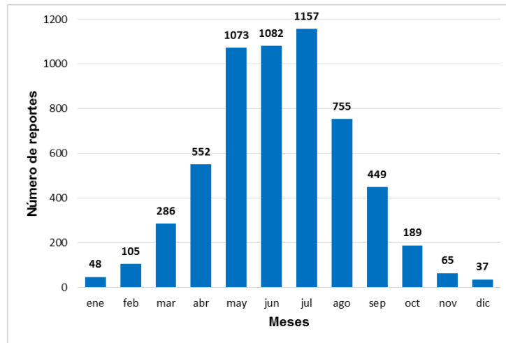
Figura 2. Distribución mensual de reportes de Tormentas Locales Severas en Cuba entre los años 1980 hasta el 2020.
