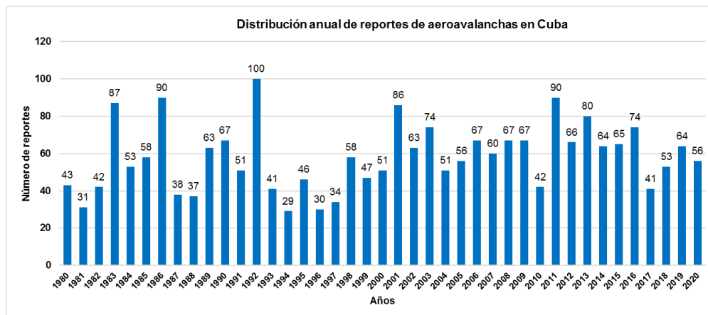
Figura 9. Distribución anual de los reportes de aeroavalanchas en Cuba en el periodo 1980 - 2020.
