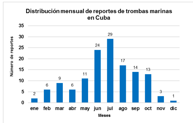
Figura 16. Distribución mensual de los reportes de tromba marina en Cuba en el periodo 1980 - 2020.
