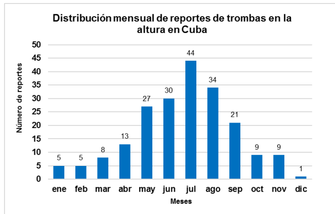
Figura 14. Distribución mensual de los reportes de tromba en altura en Cuba en el periodo 1980 -2020.
