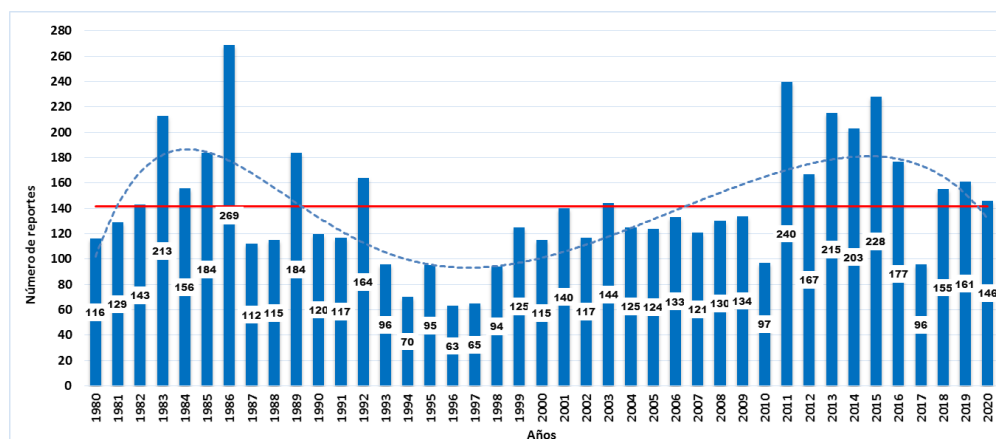
Figura 1. Distribución anual de reportes de Tormentas Locales Severas en Cuba entre los años 1980 y 2020.
