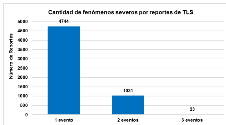
Figura 5. Cantidad de eventos severos por reporte de Tormentas Locales Severas en Cuba entre los años 1980 y 2020.
