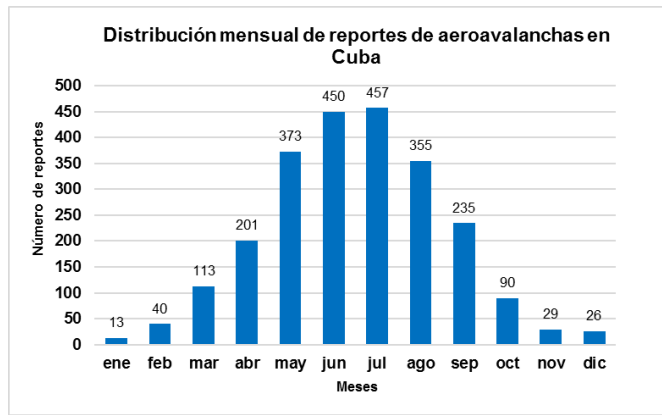
Figura 10. Distribución mensual de los reportes de aeroavalanchas en Cuba en el periodo 1980 - 2020.
