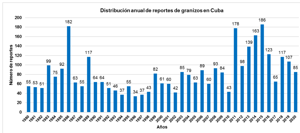
Figura 7. Distribución anual de los reportes de granizos en Cuba para el periodo 1980 -2020.
