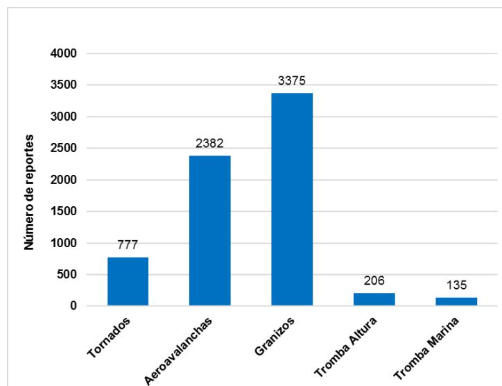
Figura 6. Cantidad de reportes para cada fenómeno severo en Cuba entre los años 1980 y 2020.
