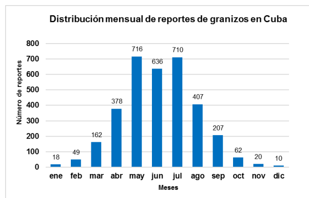
Figura 8. Distribución mensual de los reportes de granizos en Cuba para el periodo 1980 -2020.
