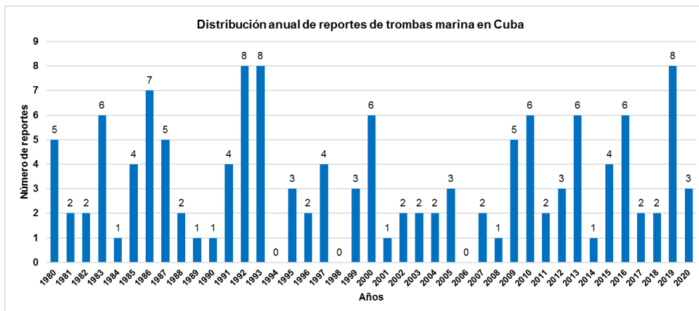
Figura 15. Distribución anual de los reportes de tromba marina en Cuba en el periodo 1980 - 2020.
