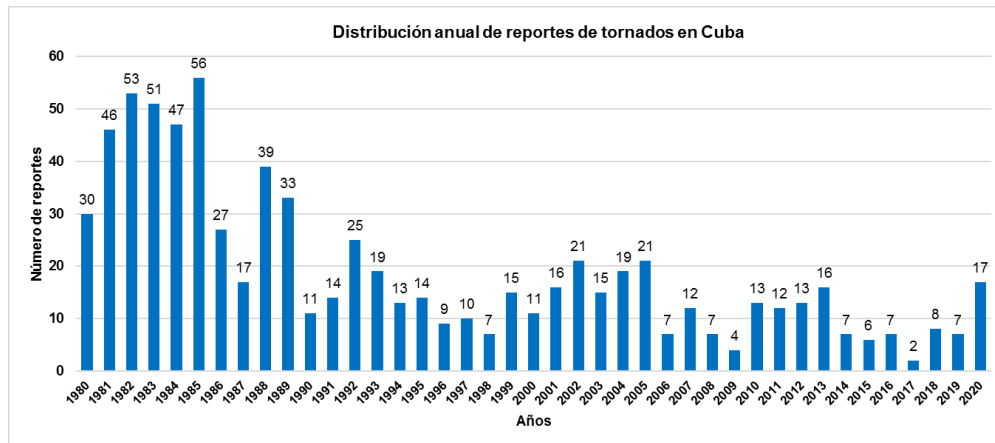
Figura 11. Distribución anual de los reportes de tornado en Cuba en el periodo 1980 - 2020.
