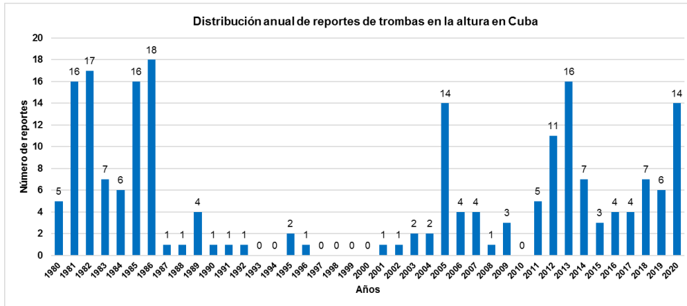
Figura 13. Distribución anual de los reportes de tromba en altura en Cuba en el periodo 1980 - 2020.
