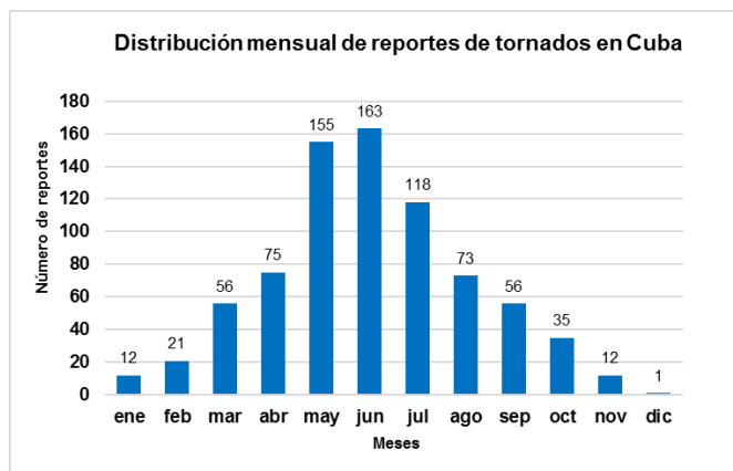
Figura 12. Distribución mensual de los reportes de tornado en Cuba en el periodo 1980 - 2020.
