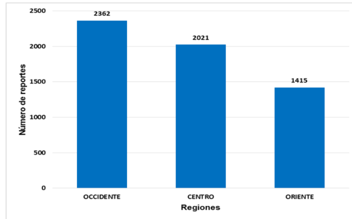
Figura 4. Distribución de reportes de Tormentas Locales Severas por regiones en Cuba entre el periodo 1980 y 2020.
