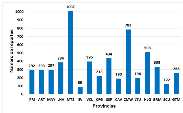
Figura 3. Distribución de reportes de las Tormentas Locales Severas por provincias en Cuba en el periodo entre 1980 y 2020.
