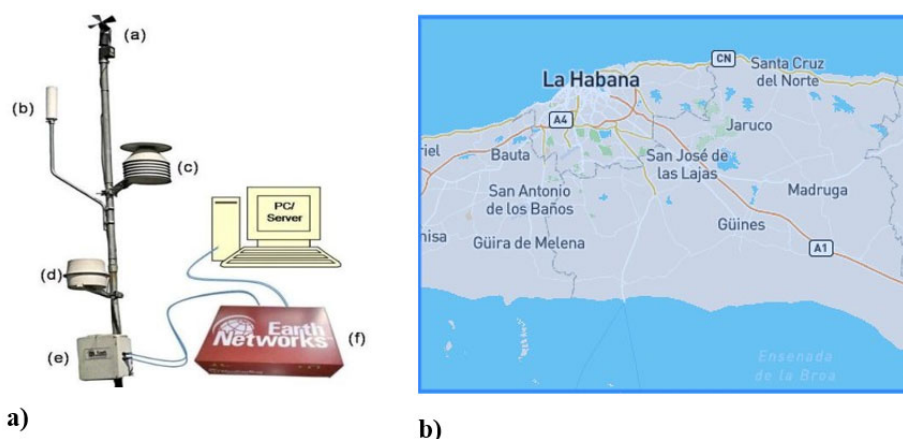
Figura 2.2 a . (Izquierda) Earth Networks, detector total de rayos e instrumentos meteorológico. a) Sensor de velocidad y dirección del viento, b) sensor integrado de detección de rayos en la nube (IC) y de nube a tierra (CG), c) refugio el sensor, d) lluvia Gauge, e) Caja de Control remoto de descargas, f) Dispositivo de Red, Midya, 2018. Figura 2.2 b (Derecha) Área que se utilizó para extraer las descargas eléctricas
