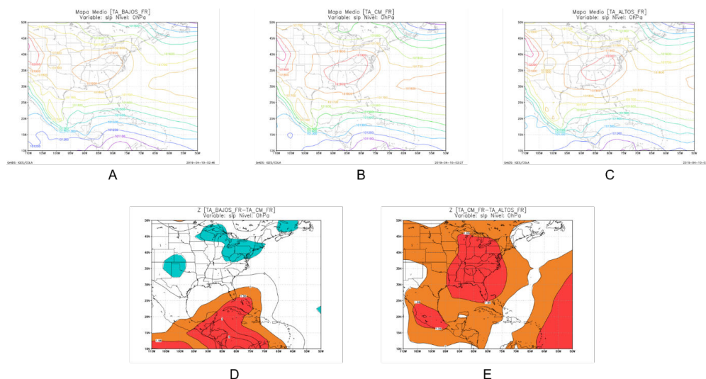
Figura 8. Configuraciones medias de presión a nivel medio del mar para los frentes reversinos de los trimestres bajos (A), normales (B) y altos (C). Mapas de significación entre trimestres bajos y normales (D) y trimestres altos y normales (E)
