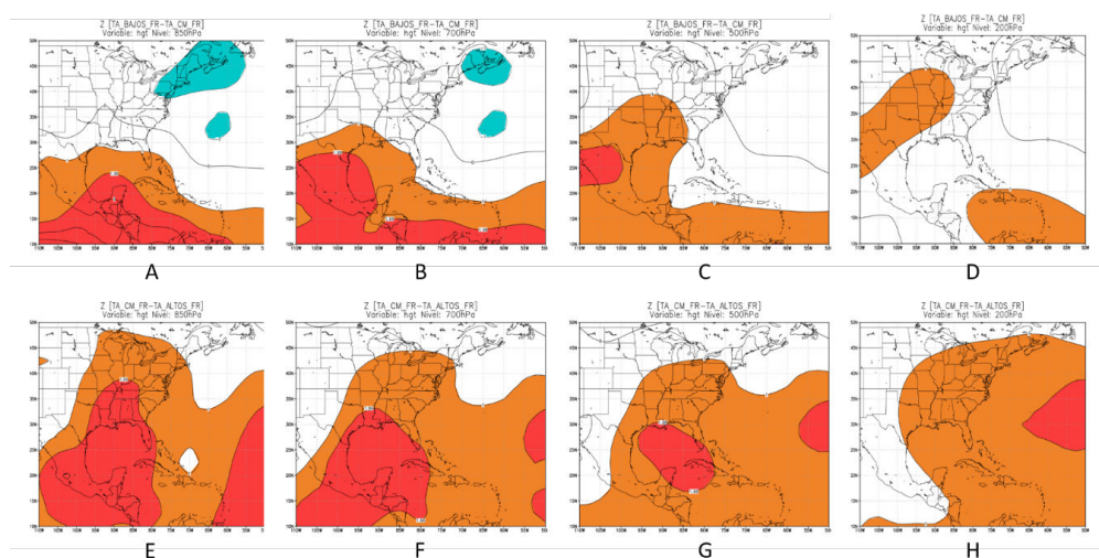
Figura 9. Mapas de significación del campo de altura geopotencial de los frentes reversinos entre trimestres normales y bajos para los 850 hPa (A), 700 hPa (B), 500 hPa (C) y 200 hPa (D); y entre trimestres altos y normales para los 850 hPa (E), 700 hPa (F), 500 hPa (G) y 200 hPa (H)
