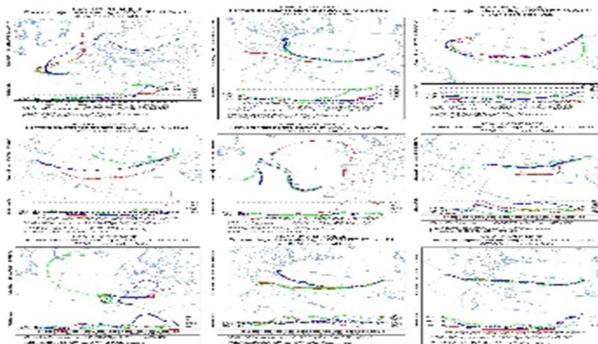
Figura 4. Salida del modelo de trayectoria Hysplit cada 10 días (a partir del 19 de septiembre de 2021)
