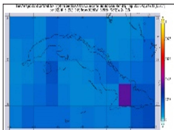
Figura 12. AOD (15 de octubre de 2022)
