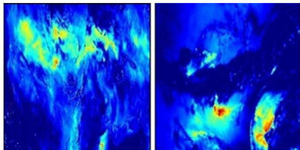
Figura 13. Nube de polvo del Sahara, Sentinel (junio 2019)
