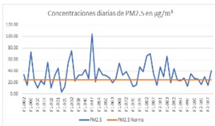
Gráfico 1. Concentraciones diarias de PM 2.5 en \mu\text{g}/\text{m}^3
