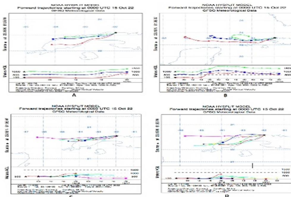
Figura 6. Salidas del modelo de trayectoria
