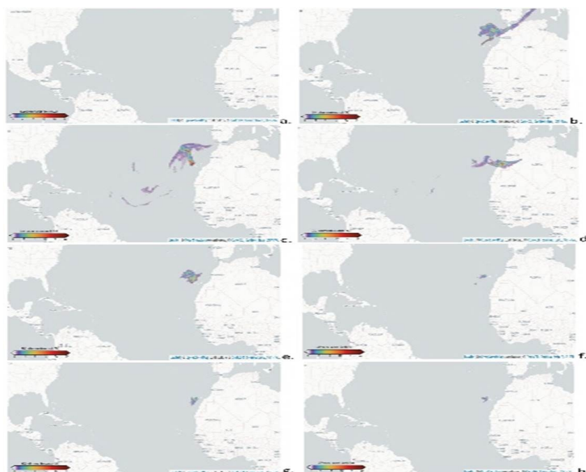
Figura 10. Densidad de la columna de dióxido de azufre expulsada por el volcán Cumbre Vieja
