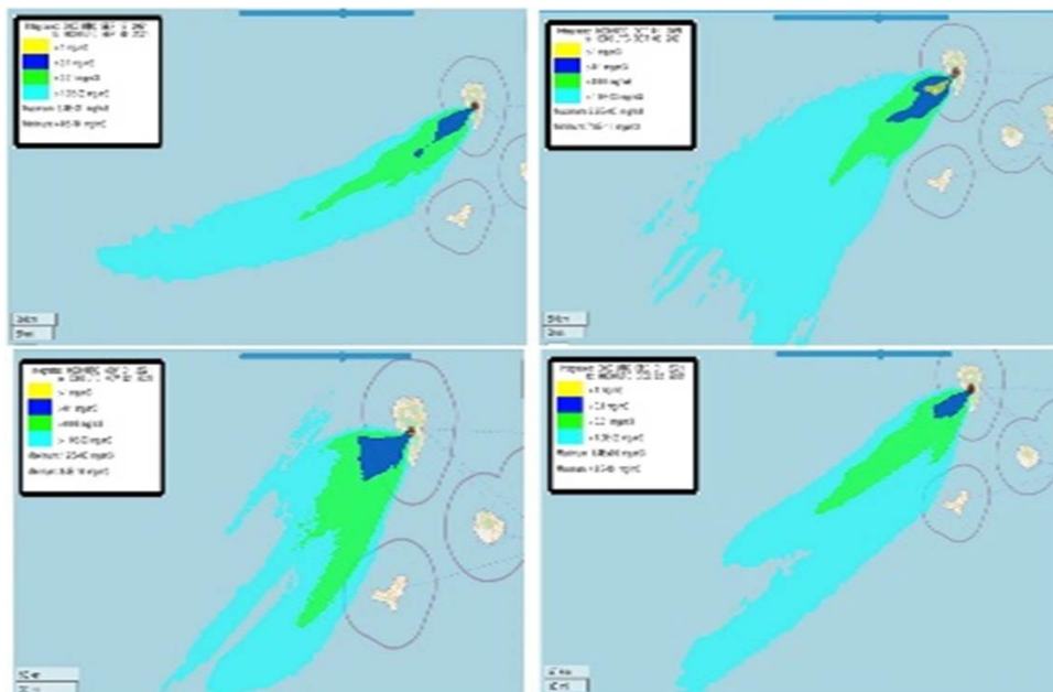
Figura 5. Salidas del modelo de dispersión
