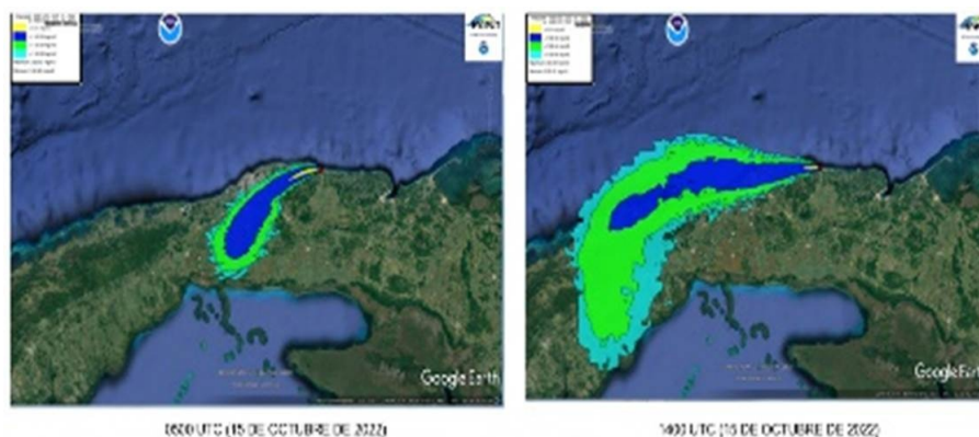
Figura 7. Salida del modelo de dispersión
