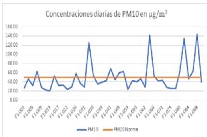
Gráfico 2. Concentraciones diarias de PM 10 en \mu\text{g}/\text{m}^3
