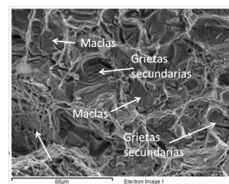
Figura 12: Fractografía Muestra B.
