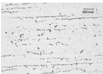
Figura 4: Micrografía muestra C (100x).
