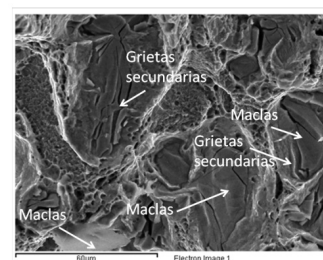
Figura 13: Fractografía Muestra C.
