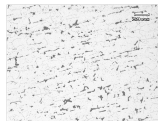
Figura 2: Micrografía muestra A (100x).
