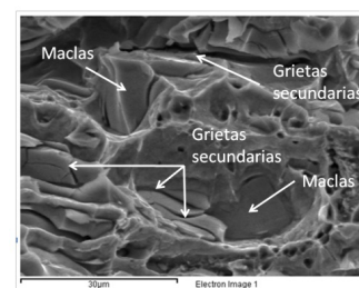
Figura 14: Fractografía Muestra D.
