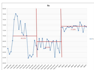
Figura 26: Resultados Fe- Zona Clara, Zona Oscura, Matriz.
