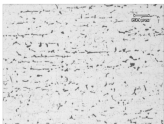
Figura 3: Micrografía muestra B (100x).
