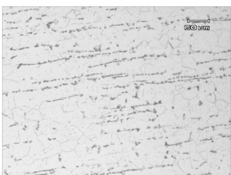
Figura 5: Micrografía muestra D (100x).
