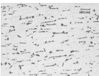
Figura 6: Micrografía muestra E (100x).
