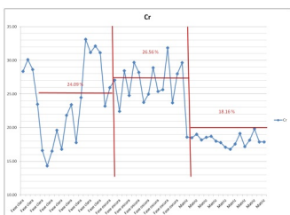
Figura 27: Resultados Cr- Zona Clara, Zona Oscura, Matriz.
