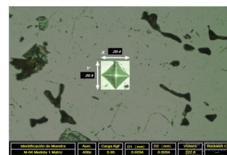
Figura 8: Medición de dureza en la fase de la muestra B.
