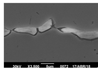
Figura 21: Micrografía de muestra C evaluada mediante back scattered electron (3500x).
