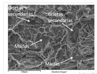
Figura 11: Fractografía Muestra A.
