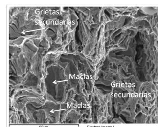
Figura 15: Fractografía Muestra E.
