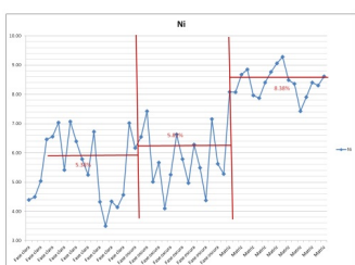
Figura 28: Resultados Ni- Zona Clara, Zona Oscura, Matriz.
