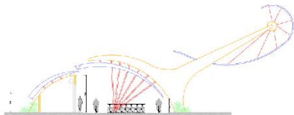
Figura 8: Biciestación Plaza de Toros-Metro Valencia, Arq. J.M Fernández
