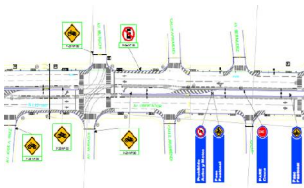
Figura 6: Eje 4. Tramo de Av. Libertador enlace Plaza de Toros, esquema funcional
