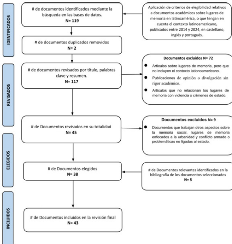
Figura 1. Diagrama PRISMA
