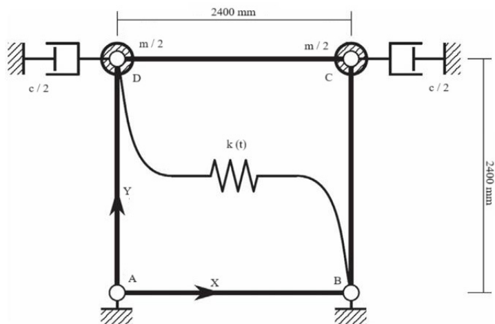
Figura 9. Composición del modelo de elementos finitos simplificado propuesto por Boundad et al. [39]
