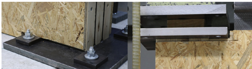
Figura 5. Espacios libres entre el panel de revestimiento y los andajes esquineros, tomada de Sadeghi et al. [20]
