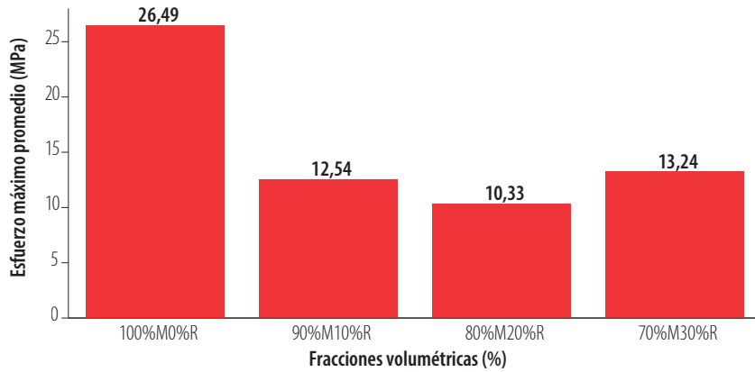
Figura 4. Comparación entre esfuerzos máximos a tracción.
