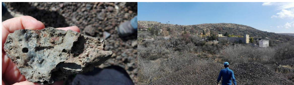
Figura 2. Muestra “de mano” (izquierda). Depósito de escorias muestreados en Monte Caldera (derecha).
