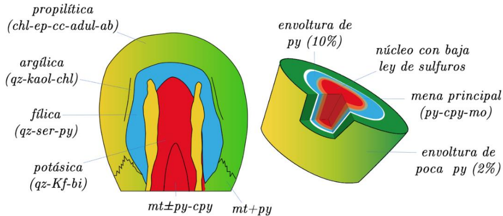
Figura 2. Modelo tradicional de los depósitos tipo pórfido de cobre, mostrando el zonamiento lateral de la alteración (izquierda) y de los minerales de mena (derecha). Chl (clorita), Ep (epidota), cc (calcocita), adul (adularia), ab (albita), qz (cuarzo), kaol (kaolinita), ser (sericita), py (pirita), Kf (feldespato potásico), bi (biotita), cpy (calcopirita), mo (molibdenita) y mt (montmorillonita).
