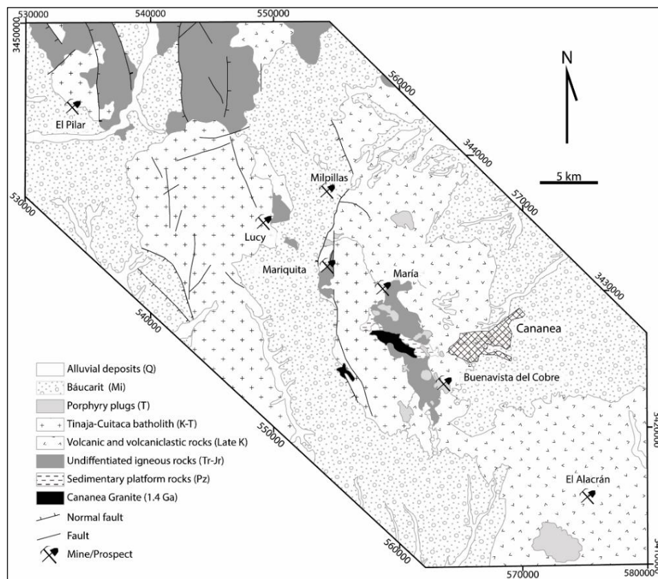
Figura 4. Mapa geológico del distrito de Cananea mostrando la distribución de las principales unidades litológicas, rasgos estructurales y la ubicación de los depósitos de pórfido de cobre (Tomado de [8]).
