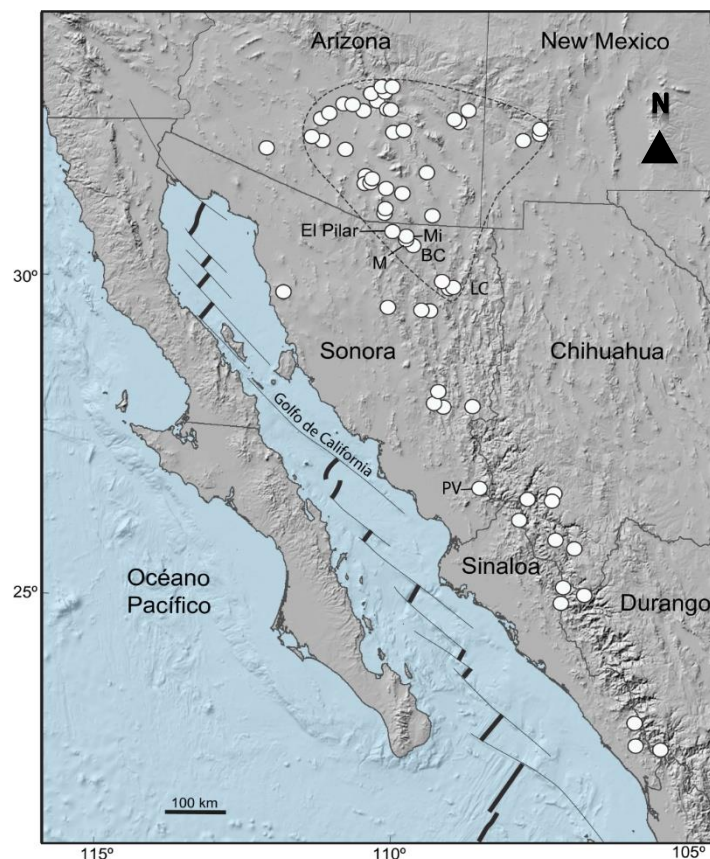
Figura 1. Localización de la porción principal del cinturón de pórfidos de cobre del suroeste de Norteamérica, mostrando los depósitos más importantes (círculos blancos). La línea punteada limita la zona del gran clúster. BC: Buenavista del Cobre; LC: La Caridad; M: María; Mi: Milpillas; PV: Piedras Verdes.
