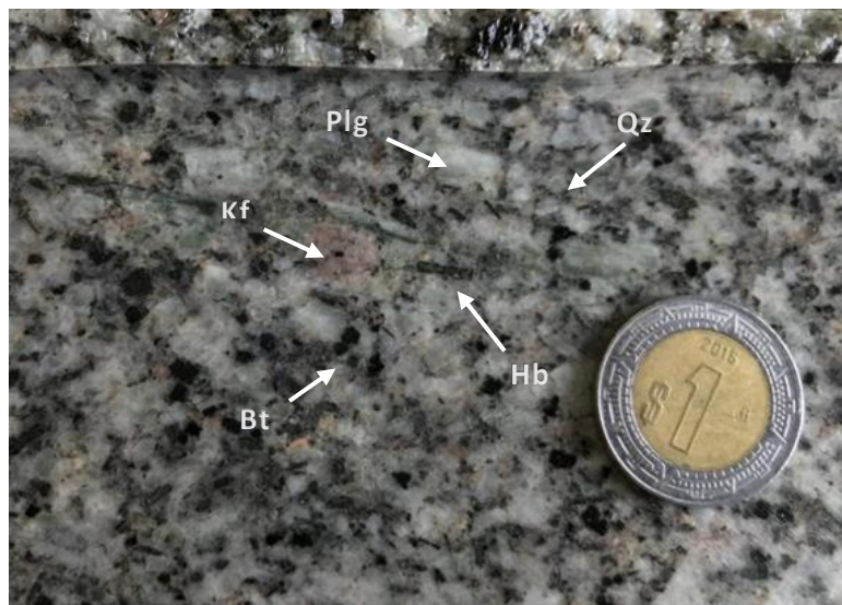
Figura 6. Fotografía del intrusivo cuarzomonzonítico tomada de una muestra de núcleo de barrenación, mostrando un aspecto de la mineralogía. Plg (plagioclase); Qz (cuarzo); Kf (feldespato potásico); Hb (hornblenda); Bt (biotita).
