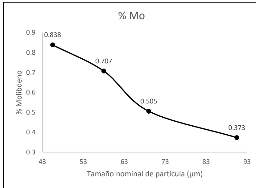
Figura 9. Análisis de FRX del molibdeno perteneciente al grupo B (Pirita molida y finos).
