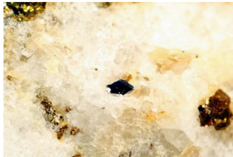
Figura 1. Molibdenita 3-R dentro de cuarzo ( \text{SiO}_2 ) y pirita ( \text{FeS}_2 ). [25]
