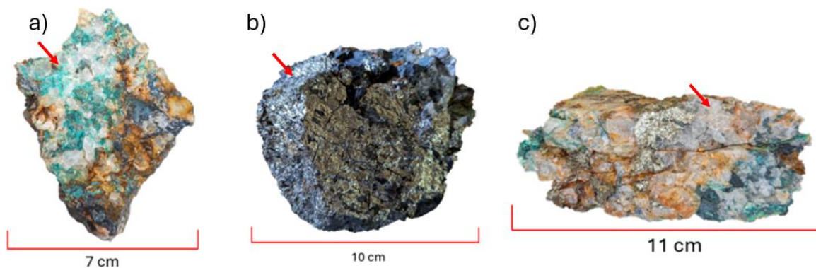
Figura 4. Trozos de mineral reducidos antes de la trituración. Se logran identificar los minerales de malaquita (a), pirita (b), y calcopirita, bornita y cuarzo (c). (fotografías propias).
