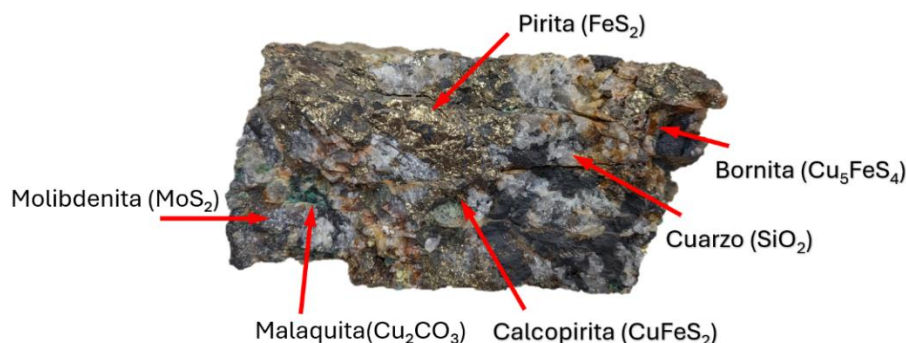
Figura 2. Mineral de Pánuco con presencia del sistema pirita-molibdenita (fotografía propia).
