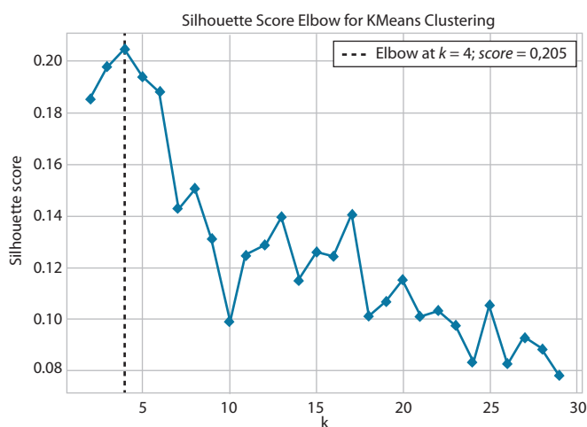
Fig. 7. Test Silhouette sobre materias.
