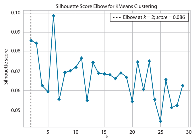
Fig. 5. Test Silhouette sobre textos.
