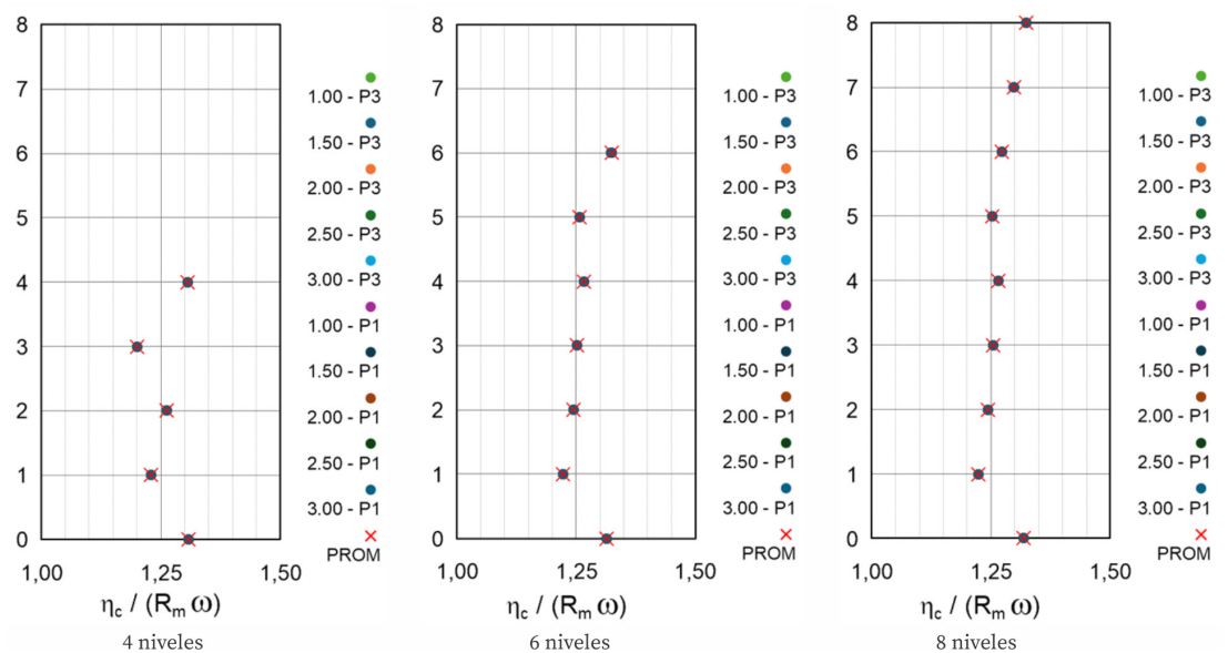
Figura 9. Factor \eta_c sin la incidencia de R_m y \omega Valores promedio de cada nivel.
