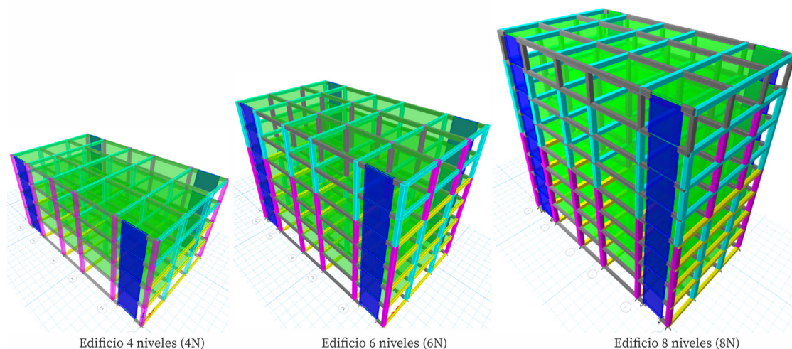
Figura 3. Edificios analizados.
