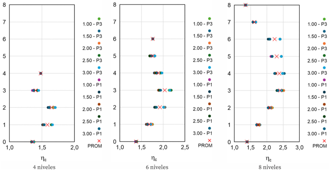
Figura 8. Factor \eta_c según IC103-II. Valores promedio de cada nivel para los distintos pórticos espaciales.
