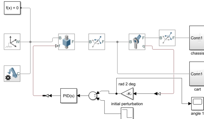
Figura 12. Implementación del control PID.
