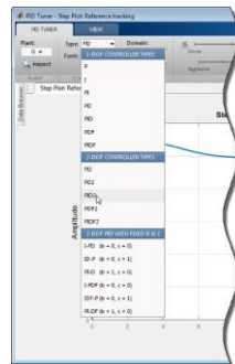
Figura 5 Aplicación PID Tuner
