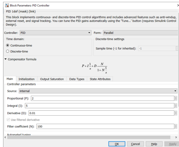
Figura 13. Parámetros del PID
