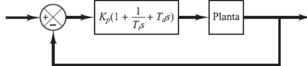
Figura 3. Control PID de la planta
