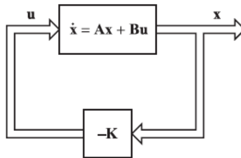
Figura 4 Sistema regulador óptimo
