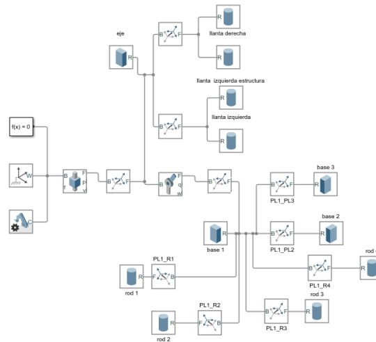
Figura 8. Modelo a bloques en Simulink®.
