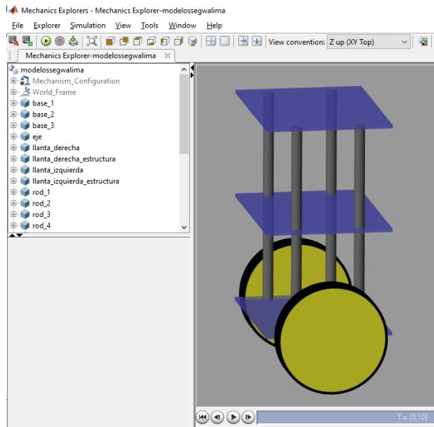
Figura 7. Modelo en Simscape™
