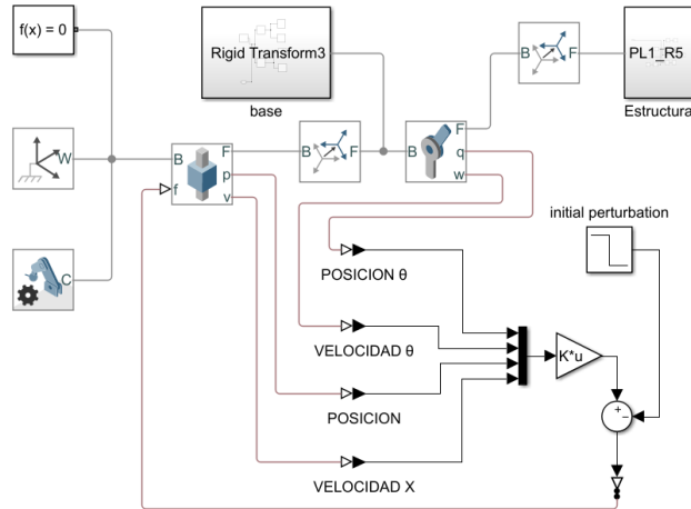
Figura 9. Implementacion del control LQR.
