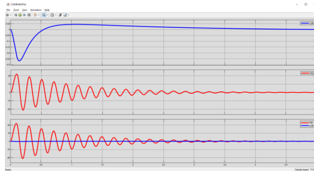
Figura 15. Comparacion entre el control PID y el LQR en el sistema con una perturbacion.
