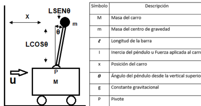
Figura 2. Sistema Péndulo Invertido sobre un Carro
