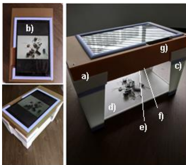
Figura 2. Dispositivo insAltech Circuit Mentor en tres diferentes vistas.
