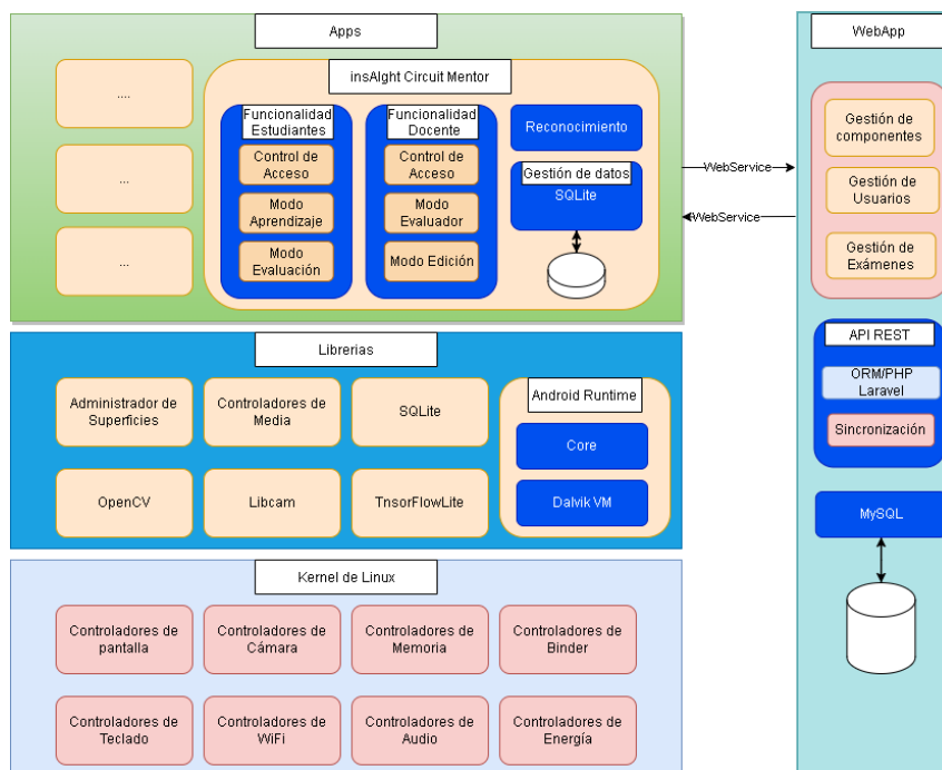
Figura 3. Arquitectura del sistema insAltech Circuit Mentor
