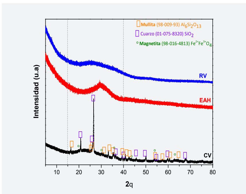
Figura 6. Diffractogramas de los residuos utilizados como precursores.
