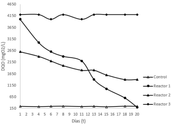
Figura 3. Medida de DQO en los reactores BK1, BK2 y BK3. Nota. Se aprecia la decadencia de la DQO en los reactores BK1 y BK2, el control es biftalato de potasio - BP y el blanco BK3.
