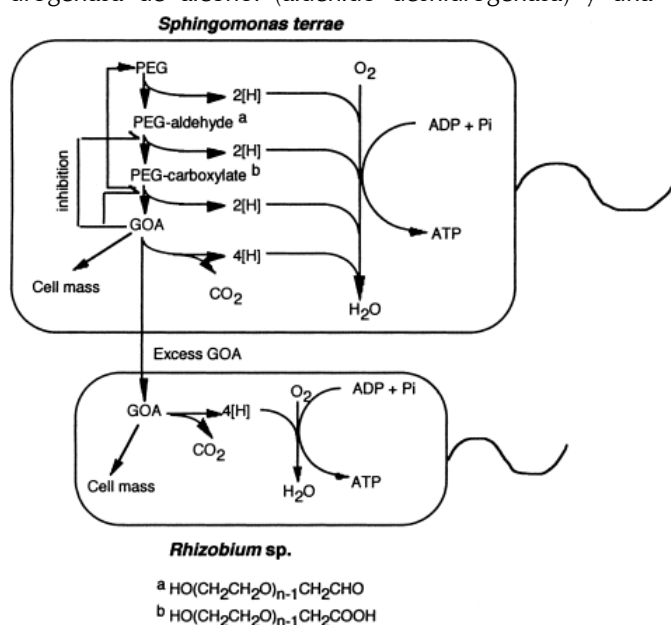
Figura 1. Mecanismo de degradación de PEG por cultivo mixto simbiótico Gram Negativo S. terrae y Rhizobium sp.
