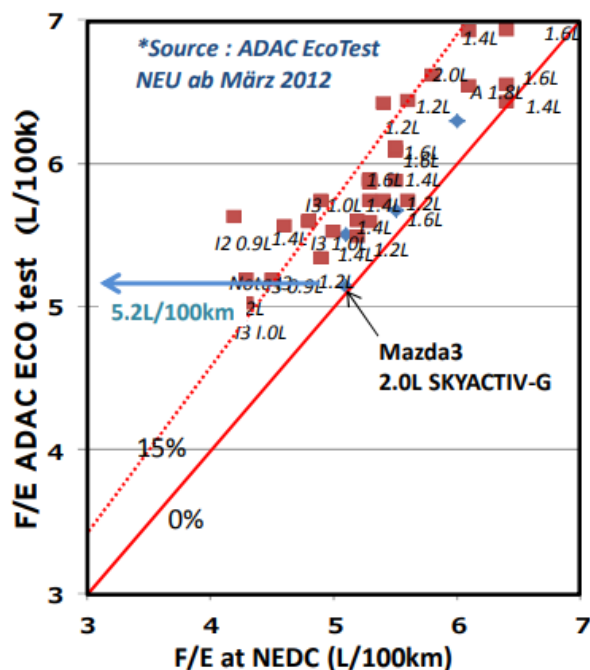
Fig. 3. Comparativa de consumo de combustible de Mazda 3 con SkyActiv- G en relación a modelos de inyección indirecta
