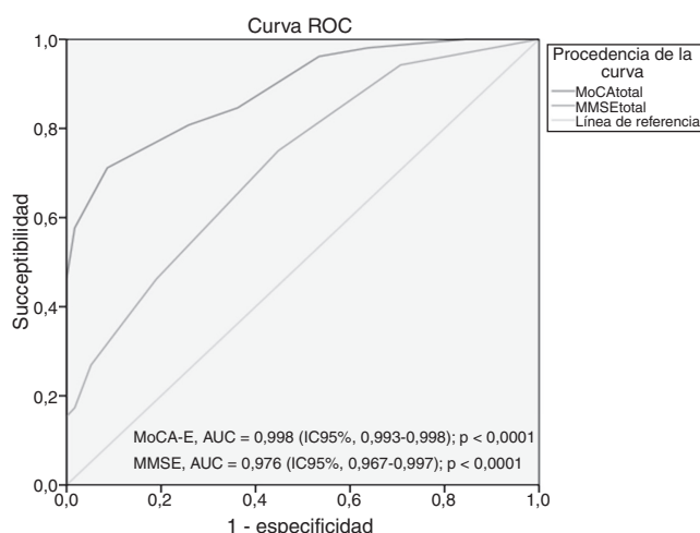
Figura 1 – Curva ROC MoCA-E frente a MMSE en DCL. DCL: deterioro cognitivo leve. AUC: área bajo la curva ROC; IC95%: intervalo de confianza del 95%.
