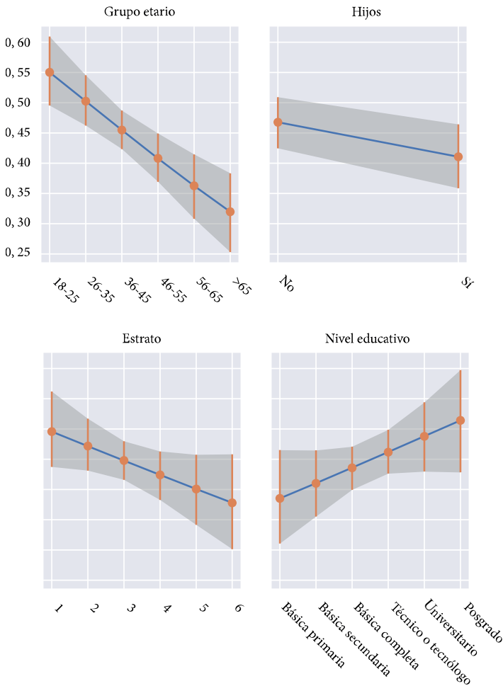
Gráfico 5. Probabilidad estimada de votar por Gustavo Petro para diferentes características socioeconómicas, calculada para las demás variables en su valor medio
