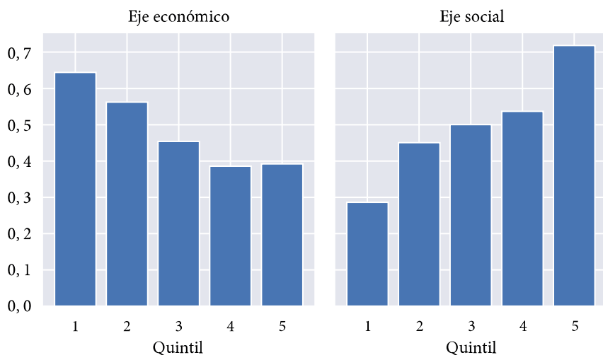
Gráfico 7. Porcentaje de personas que votarían por Petro según el quintil al que pertenecen en los ejes social y económico
