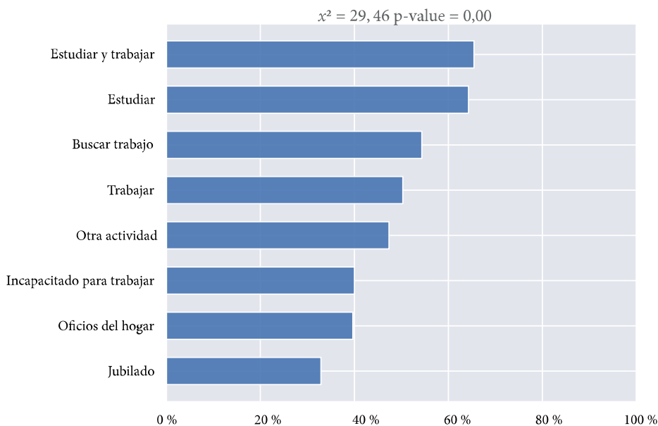
Gráfico 2. Porcentaje de personas que votarían por Petro según ocupación
