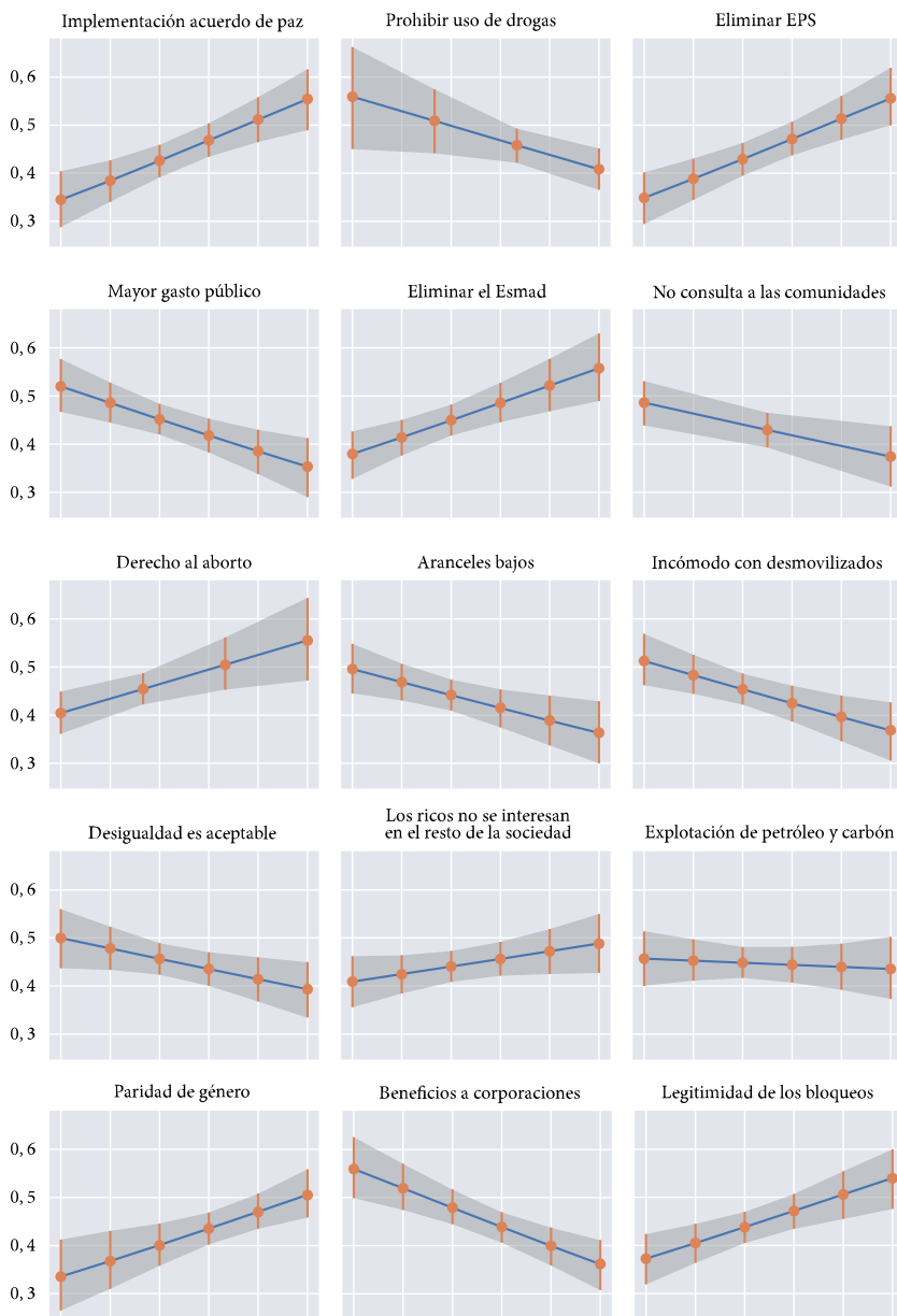
Gráfico 4. Probabilidad estimada de votar por Gustavo Petro para diferentes respuestas a los temas de opinión, calculada para las demás variables en su valor medio
