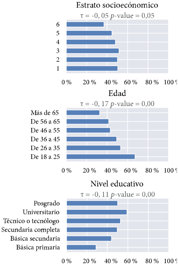
Gráfico 3. Porcentaje de personas que votarían por Petro según estrato socioeconómico, edad y nivel educativo.
