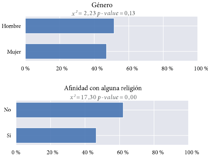
Gráfico 1. Porcentaje de personas que votarían por Petro según género y afinidad con alguna religión 4
