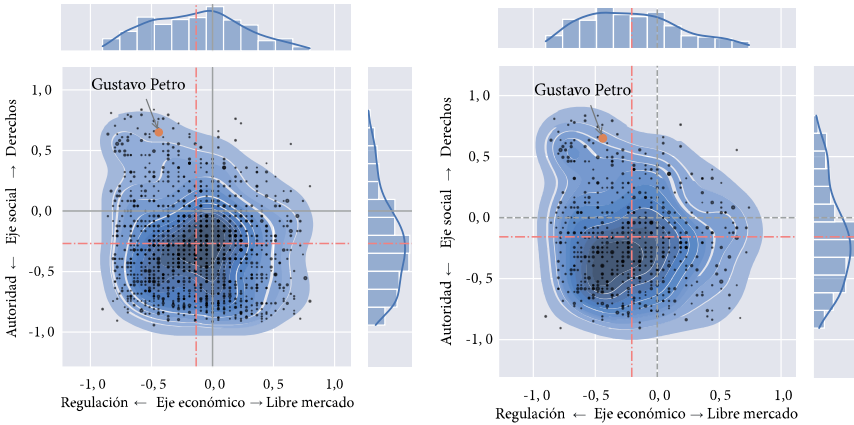
Gráfico 6. Ubicación y distribución de los encuestados en los ejes social y económico
