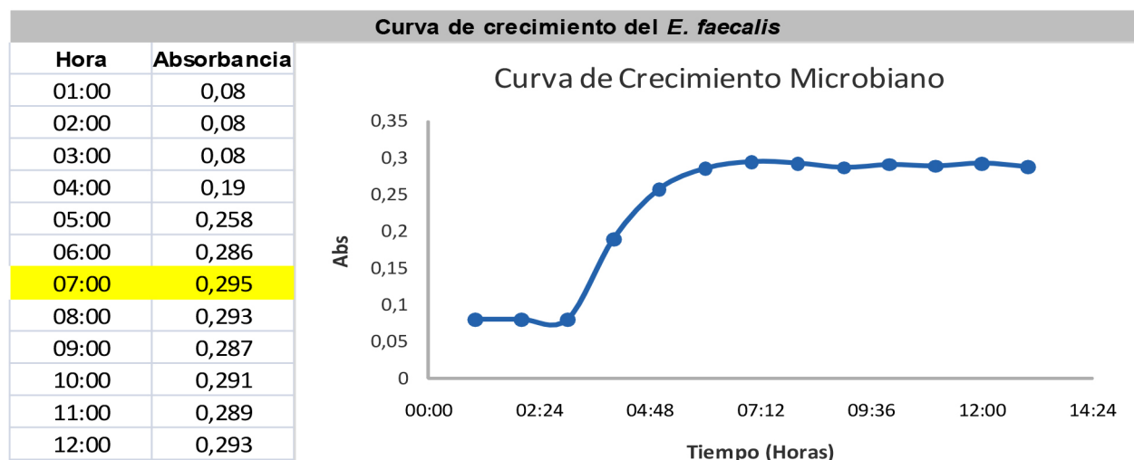
Gráfico 1. Curva de Crecimiento E. faecalis
