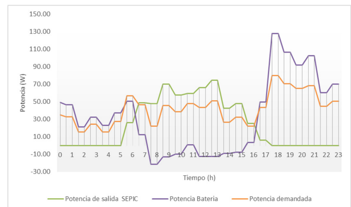
Figura 17. Comportamiento regulador, 15 de junio
