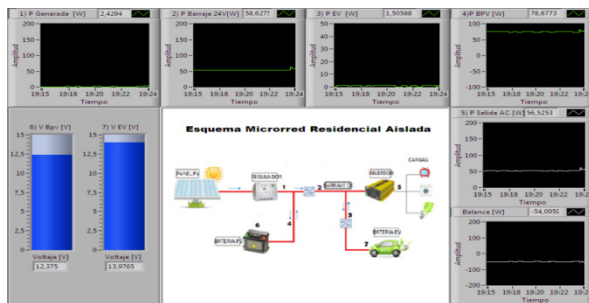
Figura 15. Panel Frontal de visualización de datos
