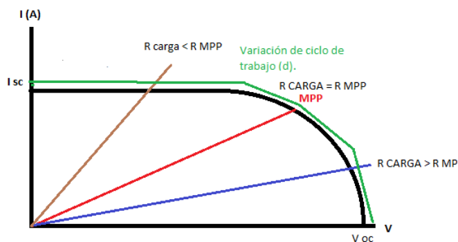
Figura 2. Zona operativa convertidor SEPIC como seguidor MPP
