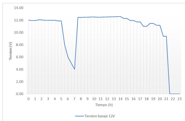
Figura 20. Comportamiento de la tensión en el barraje de 12 V, 24 de noviembre
