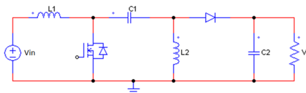
Figura 3. Topología convertidor SEPIC
