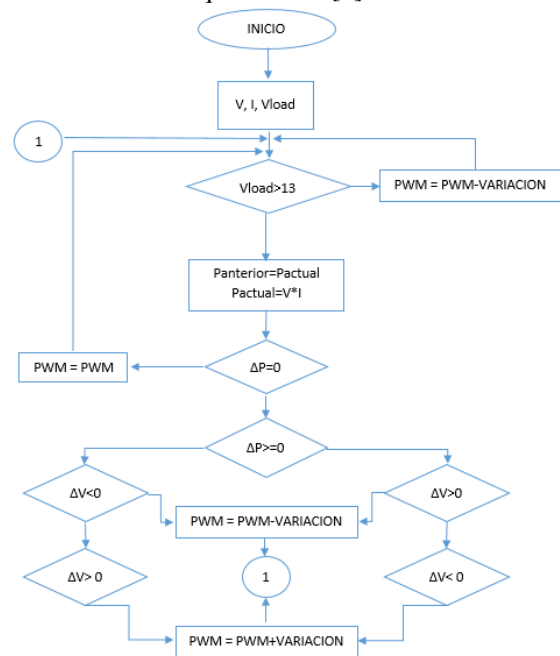
Figura 7. Algoritmo P&O
