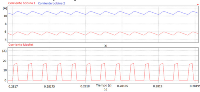
Figura 6 (a) Corrientes IL1 e IL2. (b) Corriente Mosfet con carga de 0,96 \Omega
