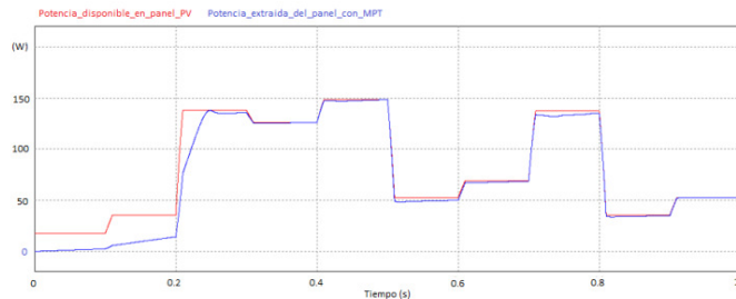
Figura 8. Curvas de potencia. Potencia disponible en el panel (Rojo). Potencia extraída del panel V \cdot I (Azul).
