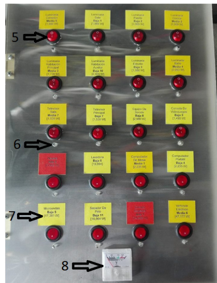
Figura 14. Panel Superior Módulo de Carga
