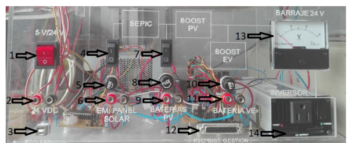
Figura 11. Panel Frontal modulo emulador de la microrred
