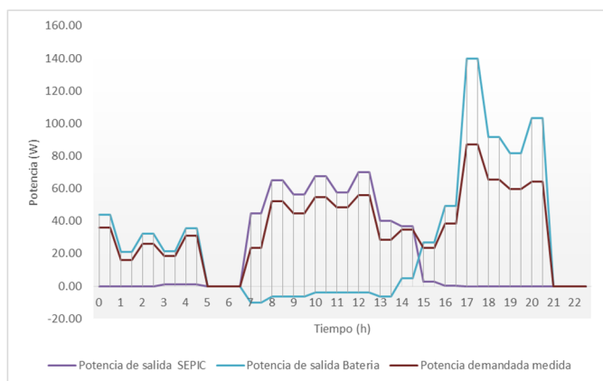
Figura 19. Comportamiento regulador, 24 de noviembre
