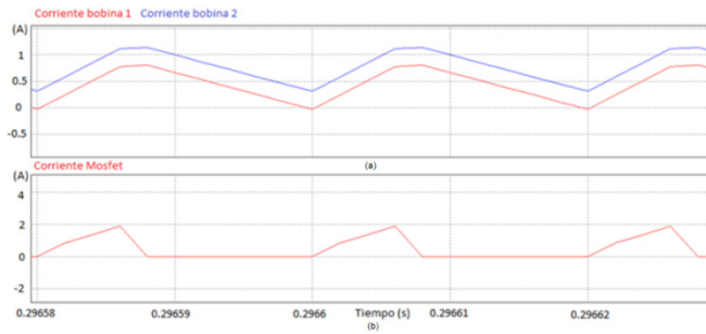
Figura 5 (a) Corrientes IL1 e IL2. (b). Corriente Mosfet con carga de 15 \Omega
