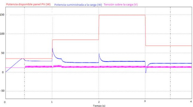
Figura 9. Curvas de potencia. Potencia disponible en el panel (Rojo). Potencia extraída del panel V \cdot I (Azul). Tensión en la carga (Rosado)
