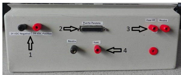
Figura 13. Panel Frontal Módulo de Carga
