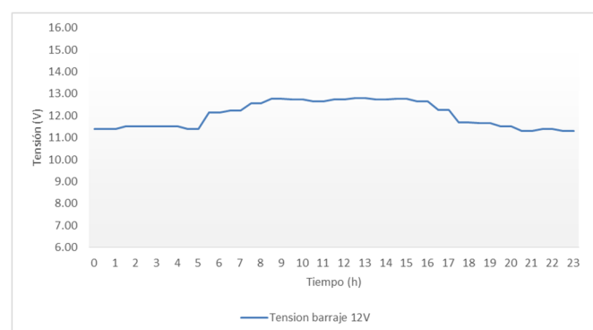
Figura 18. Comportamiento de la tensión en el barraje de 12 V, 15 de junio
