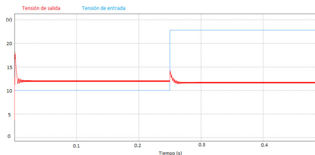
Figura 4. Tensión de salida ante variaciones en la tensión de entrada
