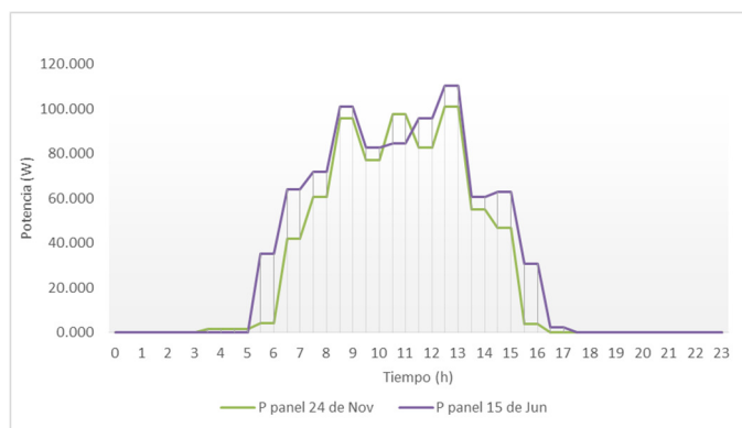
Figura 16. Curvas de potencia disponible en el panel PV
