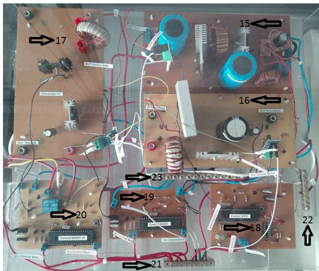
Figura 12. Nivel Superior Módulo de la microrred
