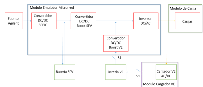
Figura 10. Plano general emulador micro red
