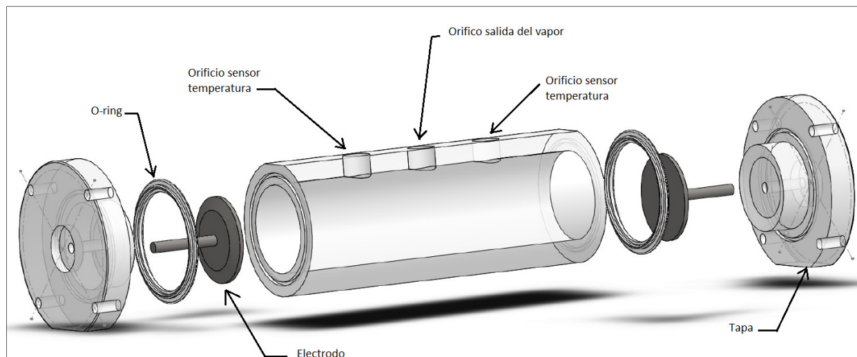
Figura 5. Despiece de la cámara de calentamiento óhmico diseñada.
