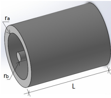
Fig 3. Configuración cilíndrica con campo eléctrico radial.
