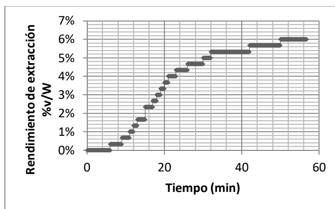
Figura 7. Hidrodestilación asistida por calentamiento óhmico
