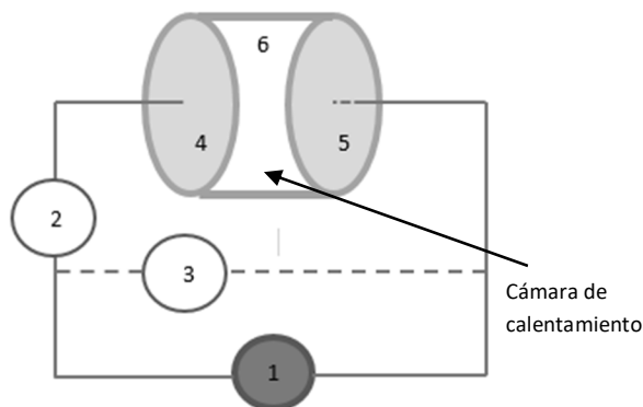
Fig 1. Configuración básica de un calentador óhmico estático.
