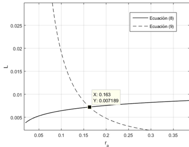
Figura 4. Solución gráfica para el diseño de la cámara 2 ( r_b = 0.2 \text{ [cm]} ).
