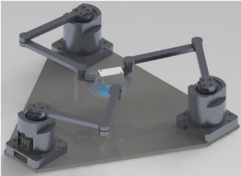
Figura 1. Manipulador 3RRR
