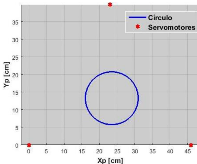
Figura 5: Trayectoria circular
