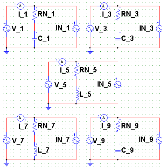
Fig. 4. Construcción de los cinco primeros equivalentes Norton del modelo de un computador personal. Fuente. Autores.
