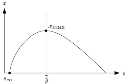
Fig. 4. Function (8).
